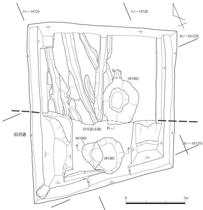
図4 調査区平面図 (S = 1/60)
