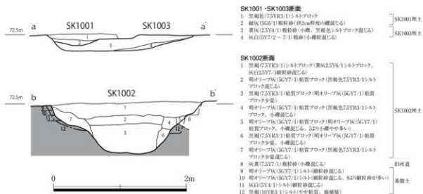
図6 SK1001～1003の断面図 (S = 1/40)
