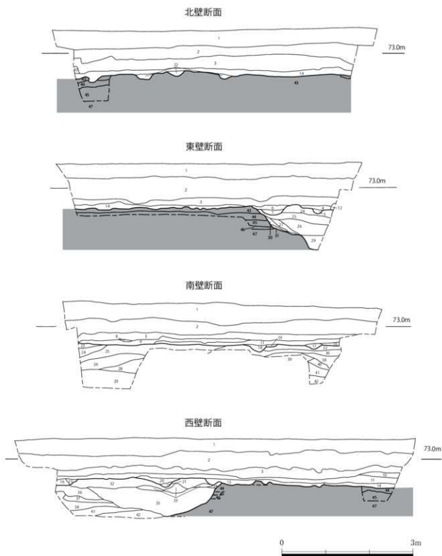
图5 调查区断面图 (S = 1/60)
