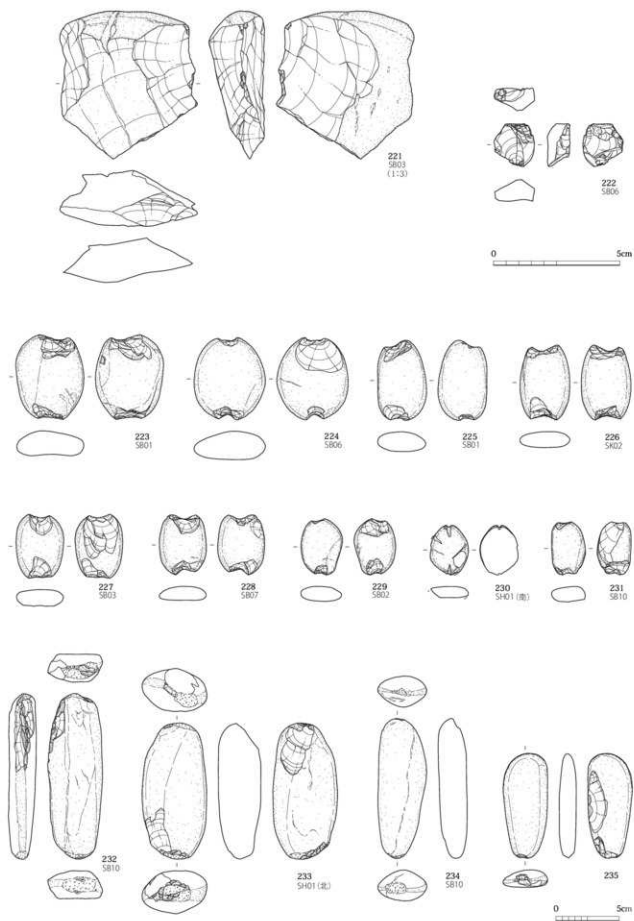
第36図 縄文石器7 (石核、石錘、敲石)
