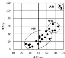
第22図 川原遺跡 石錘の重さと大きさ
