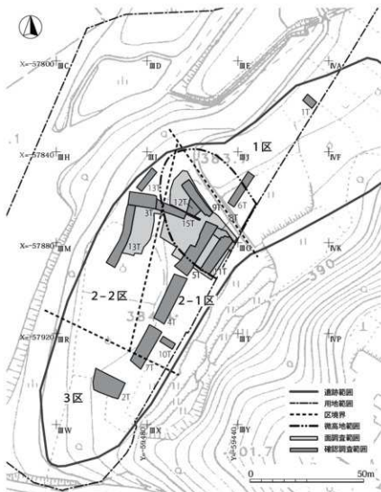
第5図 下川原遺跡トレンチ配置図
