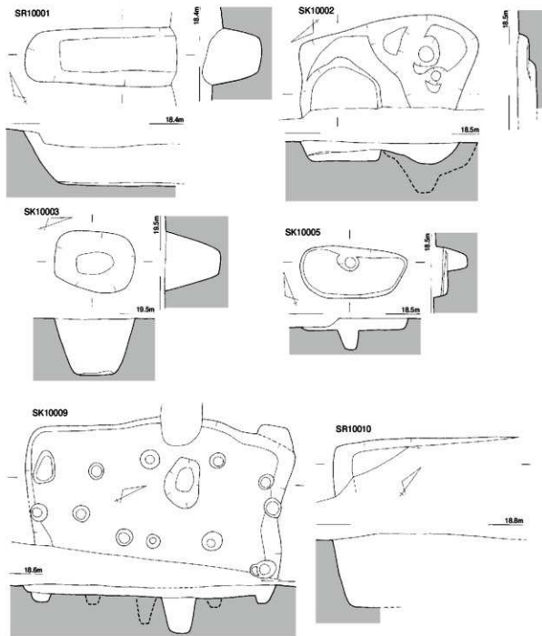
Fig.93 10区遺構実測図(1/40)
