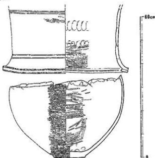
第37図 7号甕棺実測図(縮尺1/8)
