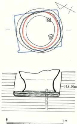
第48図 13号甕棺墓実測図 (縮尺1/20)
