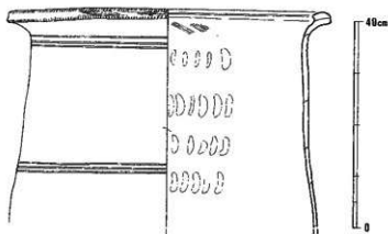
第 35 図 6号甕棺実測図 (縮尺1/8)
