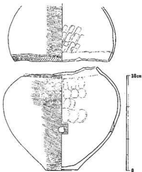
第 59 图 18号墓棺实测图 (缩尺1/6)
