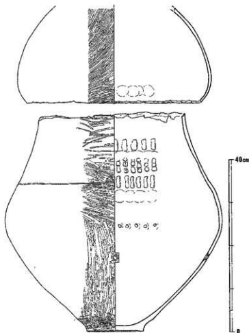
第 61 図 19号甕棺実測図 (縮尺1/6)
