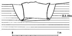
第 34 図 6号甕棺墓実測図 (縮尺1/20)
