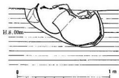
第 55 図 15号壙墓実測図 (縮尺1/20)
