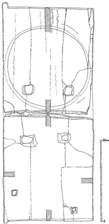
第 50 图 木器实测图 1 (缩尺 1/8)
