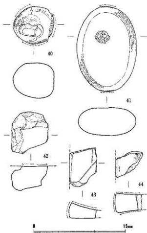
第 22 図 磨製石器・砥石実測図 4 (縮尺1/3)
