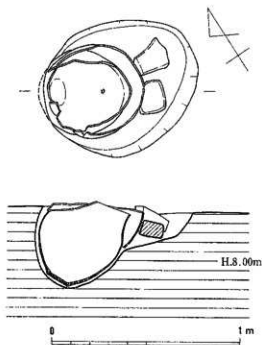
第 32 図 5号壙棺墓実測図 (縮尺1/20)
