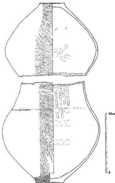
第56図 15号甕棺実測図 (縮尺1/6)
