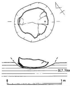
第 64 図 21号甕棺墓実測図 (縮尺1/20)
