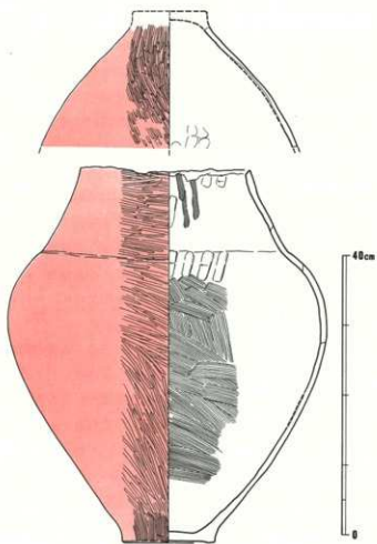
第 69 图 23号甗棺实测图 (縮尺1/6)
