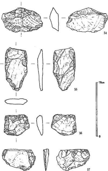
第 18 図 打製石器実測図 3 (縮尺1/2)
