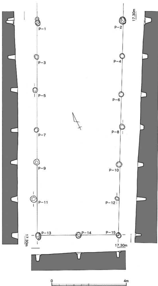
第13图 2号独立柱建物跡実測图(縮尺1/60)
