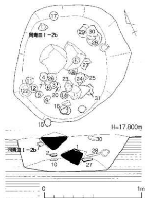
第13図 SK-05実測図(縮尺1/20)
