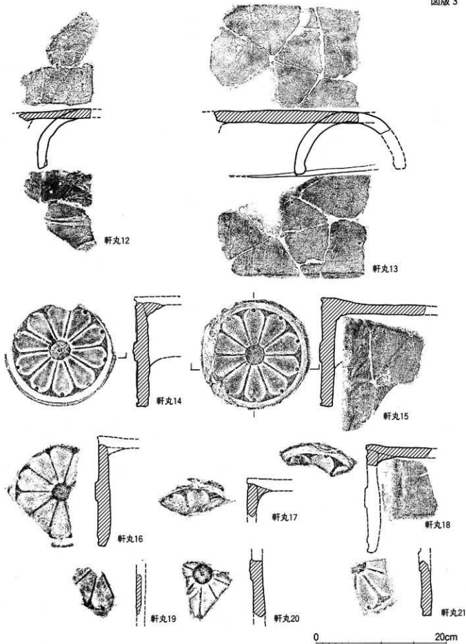
軒丸瓦A—玉縁 I 2 Za群・軒丸瓦B—行基 I 1 Za (CgまたはCh)群
