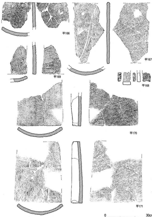
平瓦Ⅱ0 Ck群・平瓦Ⅱ0 Ck×Bj群・平瓦Ⅱ0 Ck×Cm群
