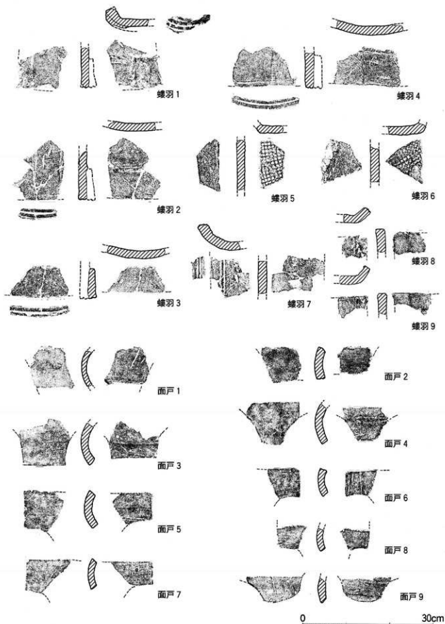
蝶羽瓦一軒平瓦AA5—平瓦Ⅱ0 Za(ⅱ)群・蝶羽瓦—平瓦Ⅱ0 Bj群・蝶羽瓦—平瓦Ⅱ3 Za群・蝶羽瓦—平瓦Ⅱ0 Za[J1e]群・蝶羽瓦—平瓦Ⅱ0 Za(ⅳ)群・切面戸瓦—玉縁 I 321 Za[J1b]群・切面戸瓦—玉縁 I 323 Za[J1b]群・切面戸瓦—行基 I 1 Za(ⅳ)群・切面戸瓦—行基 I 1 Za(xⅵⅱ)群
