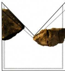
出土隅木蓋瓦復原図 (1/10)
