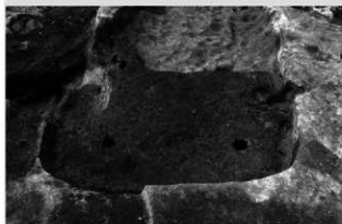
H 122 号住居址発掘
