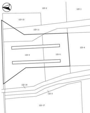
野沢城跡25 全体図(1:400)
