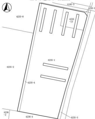
上小平遺跡5 全体図(1:500)
