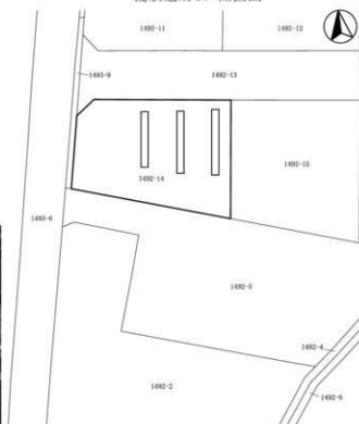
棧敷遺跡10 全体図(1:500)
