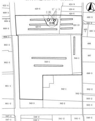
岩村田遺跡群189 全体図(1:1,000)
