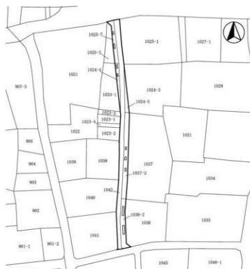
東大久保遺跡群14・白岩城跡3 全体図(1:1,200)
