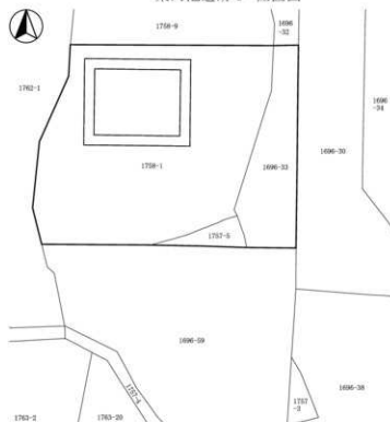
東内池遺跡 6 全体図(1:400)
