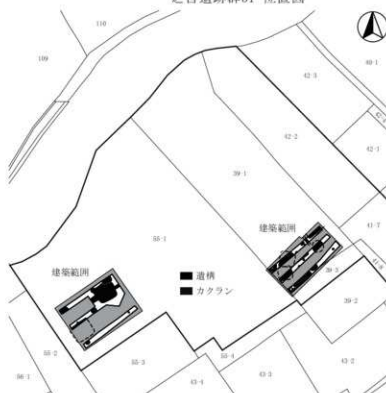
芝宮遺跡群31全体図(1:1,000)
