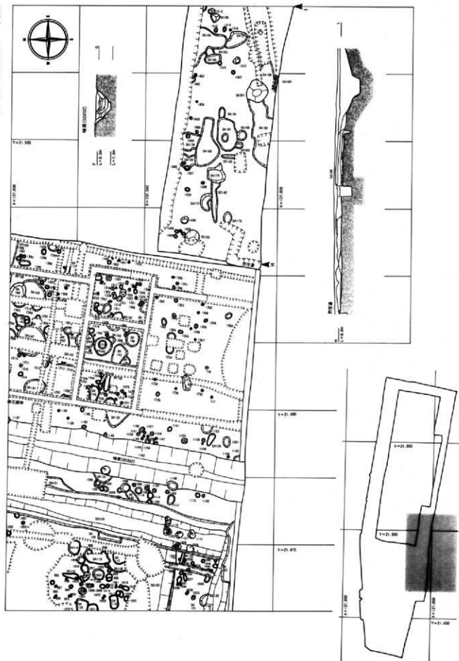
図版4 遺構配置図(4)
