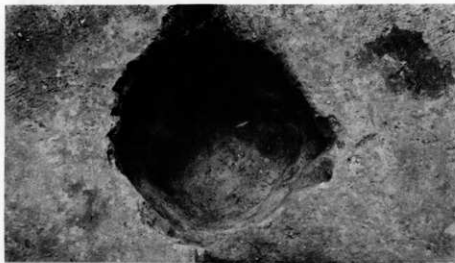
3. D-6区土塚掘り上げ後の状況（北から）
