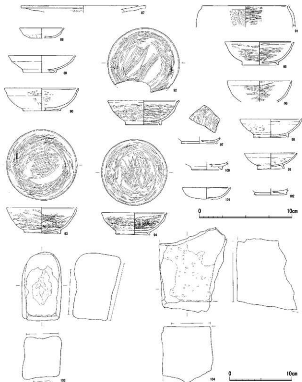
第34図 井戸4019出土遺物実測図
