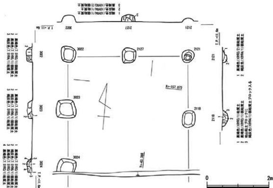
第18図 B区掘立柱建物5平面・断面図
