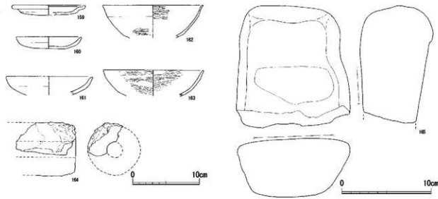
第39図 井戸6052出土遺物実測図
