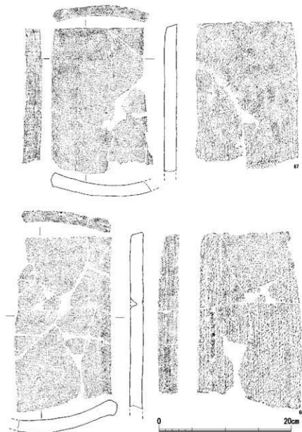
第23図 掘立柱建物6出土遺物実測図3
