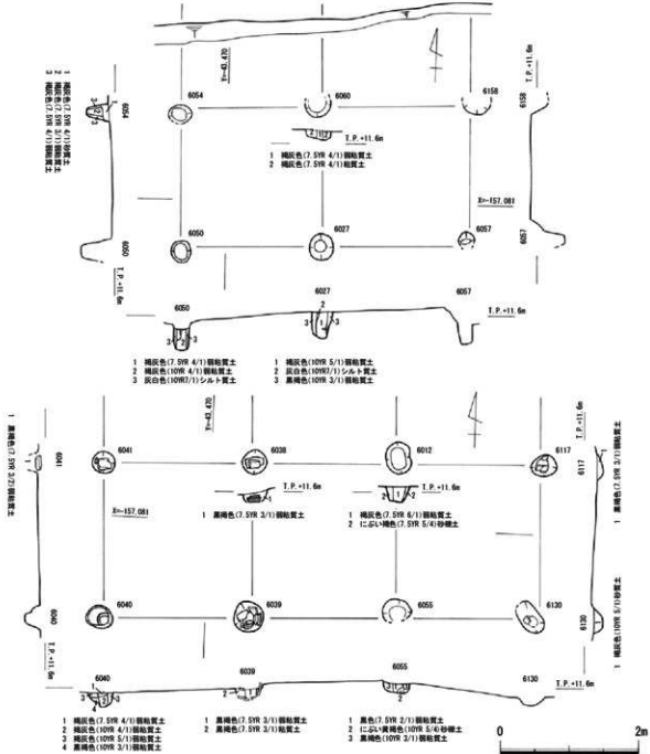
第40図 E・F・F区掘立柱建物7・8平面・断面図
