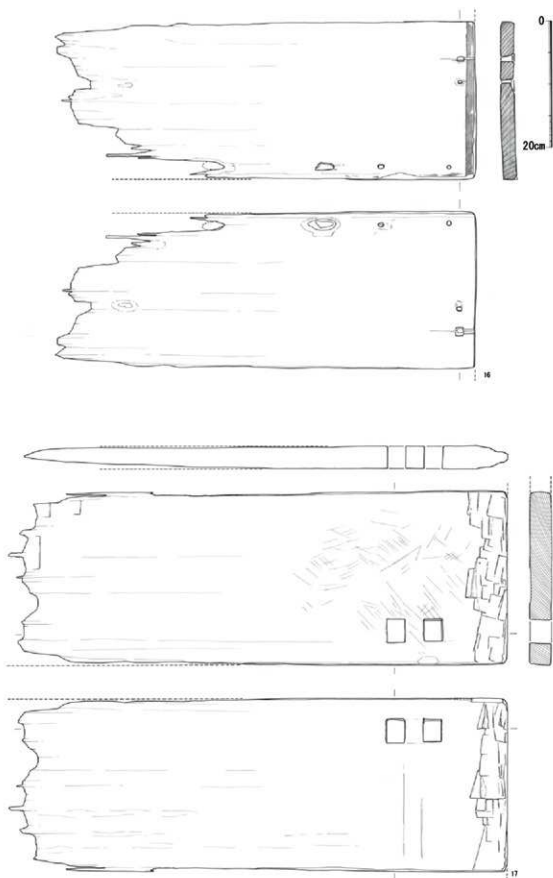
第14図 B区井戸2130井戸枠実測図6
