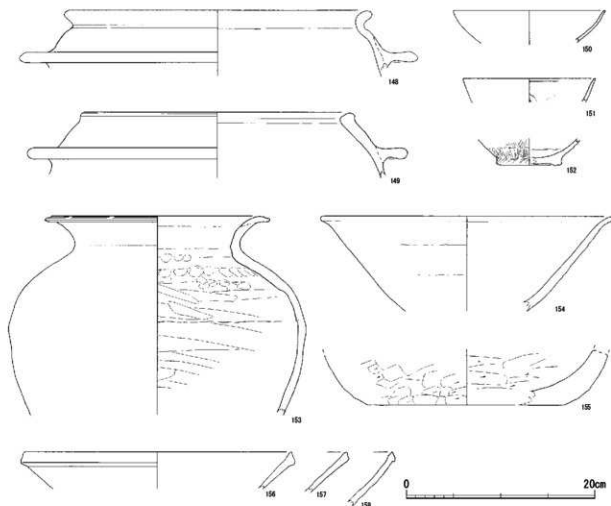
第37図 井戸5005出土遺物実測図2
