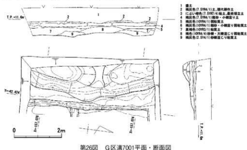
第26図 G区溝7001平面・断面図
