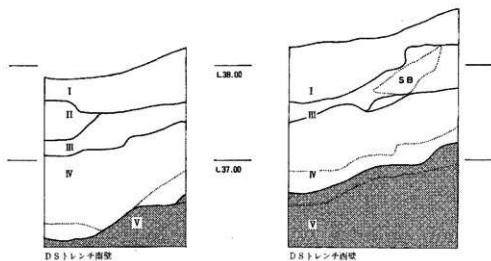
DSトレンチ南壁
