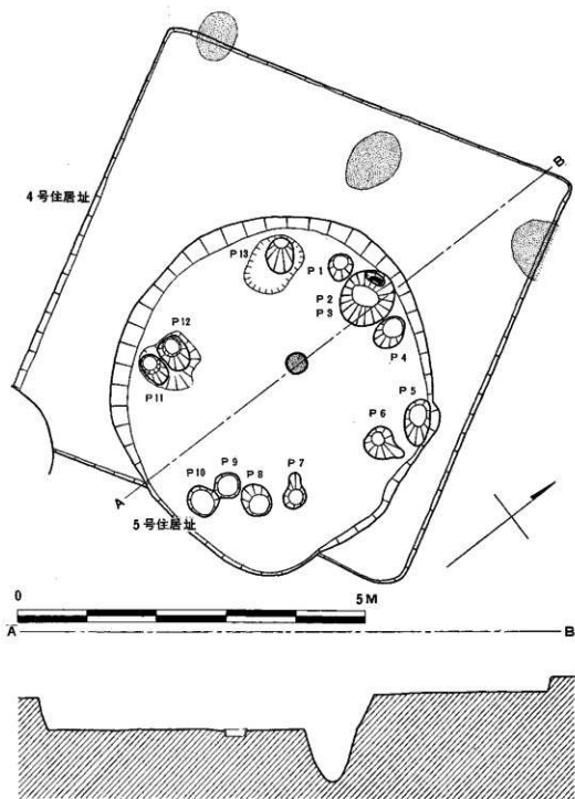
第12图 4号・5号住居址尖圆图
