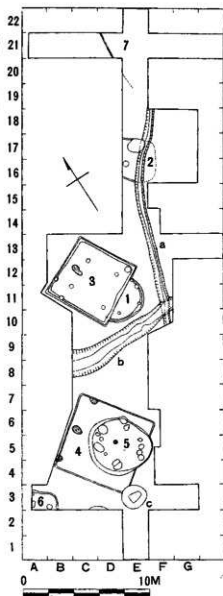
第3图 发掘区平面图
