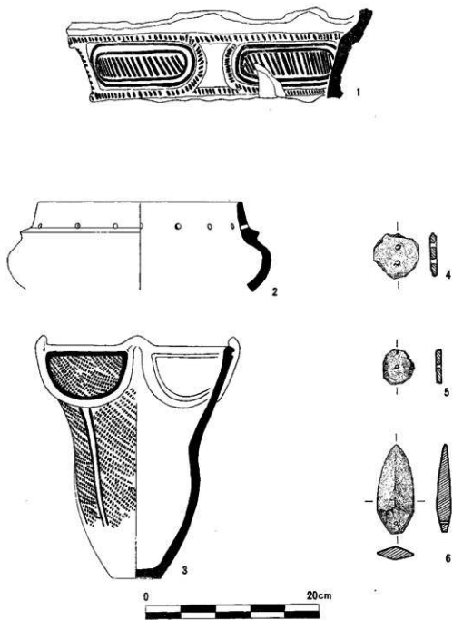
第17圖 出土遺物実測圖 1~3土器, 4~6石製模造品
