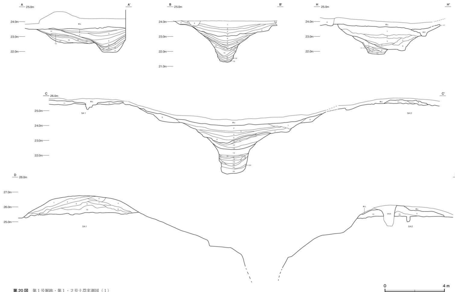
第20図 第1号堀跡・第1・2号土壘実測図(1)
