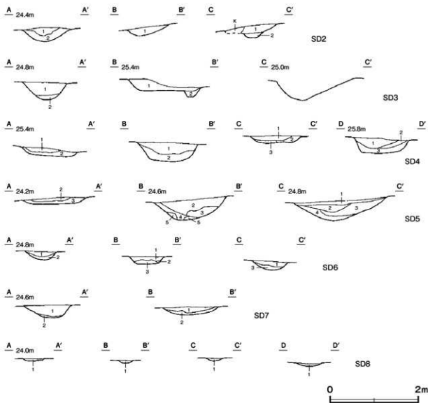
第28図 その他の溝跡実測図
