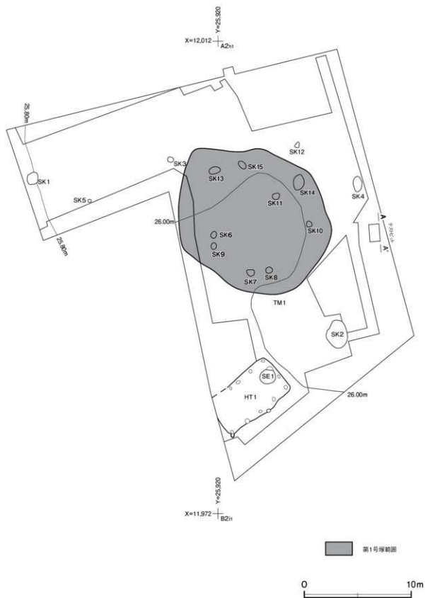
第36図 柴崎大日塚遺構全体図
