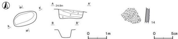
第12図 第22号土坑・出土遺物実測図
