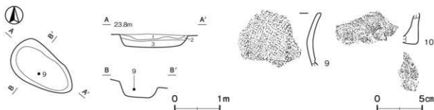
第9図 第11号土坑・出土遺物実測図
