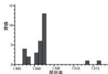
図1 火山ガラス屈折率
