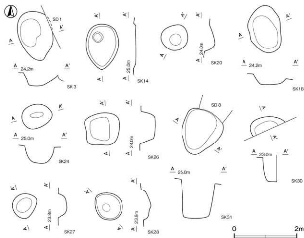
第15図 縄文時代土坑実測図(2)
