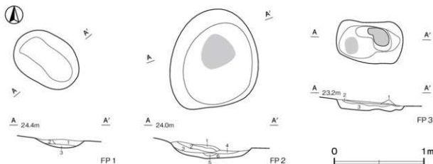
第6図 縄文時代炉跡実測図
