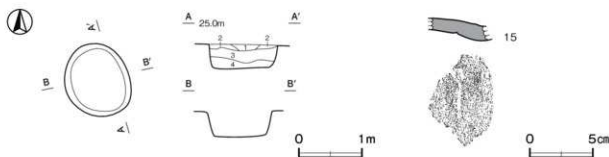
第 13 図 第 23 号土坑・出土遺物実測図
