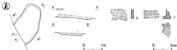
第7図 第2号土坑・出土遺物実測図
