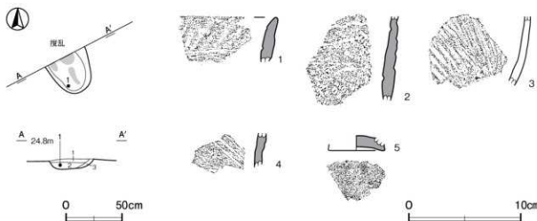
第5図 第4号炉跡・出土遺物実測図
