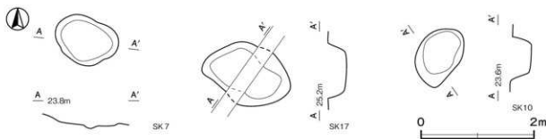
第 14 図 縄文時代土坑実測図（1）
