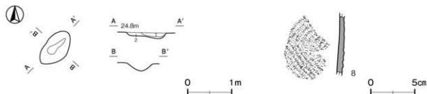
第8図 第5号土坑・出土遺物実測図
