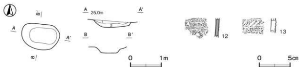
第11図 第21号土坑・出土遺物実測図
