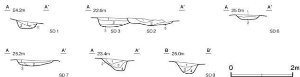
第17図 その他の溝跡実測図
