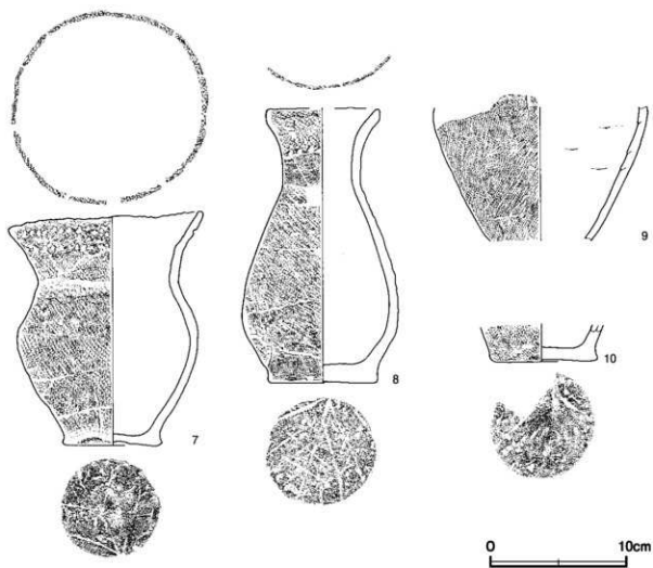
第22图 第55号竖穴建物跡・出土遺物実測図
