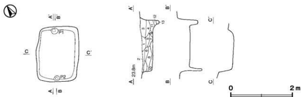
第 38 図 第 1 号堅穴遺構実測図
