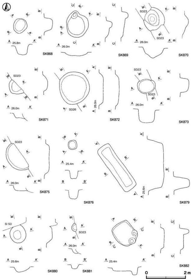
第49図 その他の土坑実測図(8)
