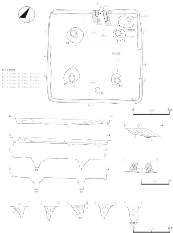
第5図 第2号竪穴住居跡(1)
