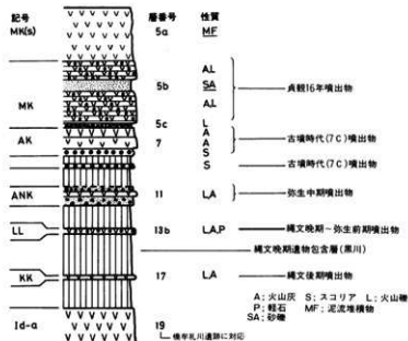
第6図 新石器後Ⅱ遺跡地質柱状図
