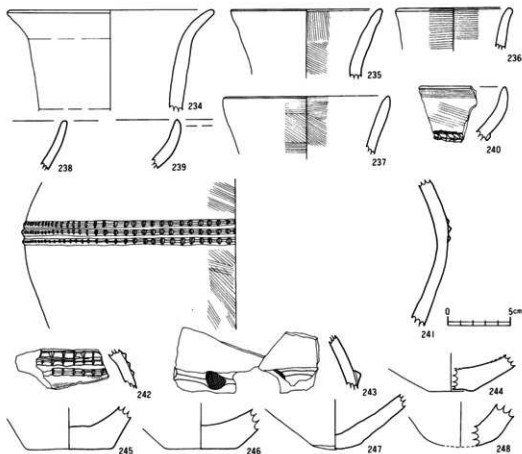
第29図 壺形土器
