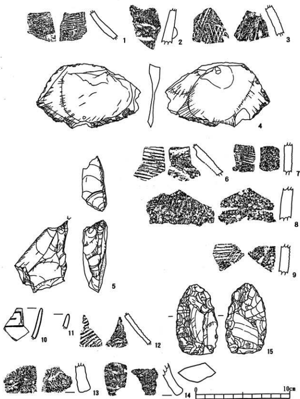
第1図 喜入町内採集遺物実測図
