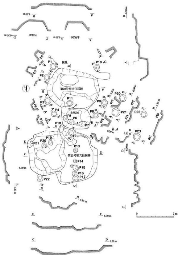
第75図 第22・23号整穴住居跡と土坑36
