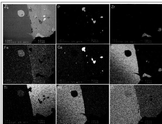
砂鉄(含チタン鉄鉱)-脈石鉱物の反射電子像(COMP)および定量分析値
