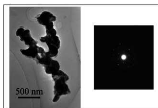
写真11 上水流遺跡出土赤色粒子TEM-EO分析
