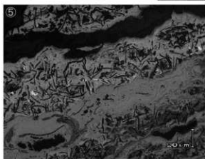
写真17 梘形鍛冶滓・鉄製品の顕微鏡組織
