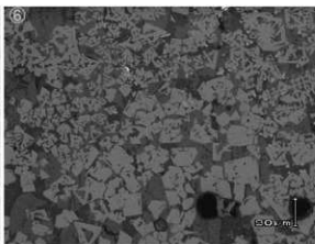
写真14 炉内滓・炉外流出滓の顕微鏡組織
