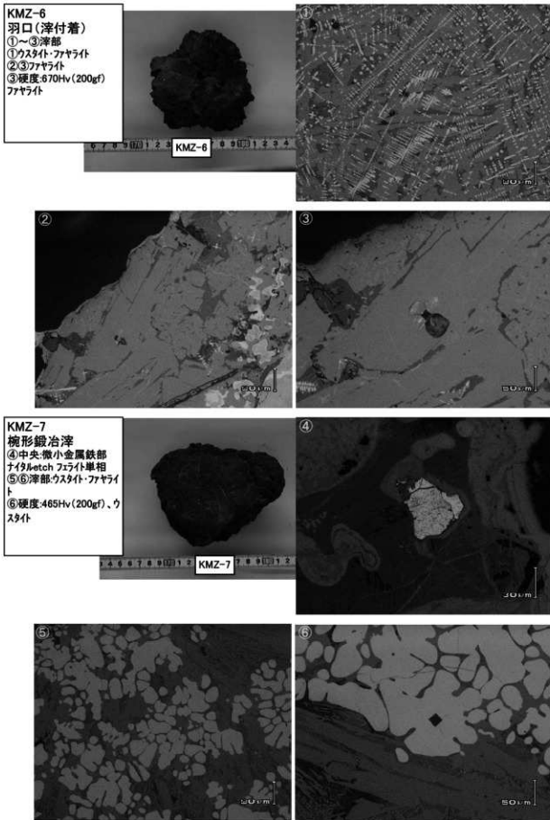
写真16 羽口 (滓附着)・椀形鍛冶滓の顕微鏡組織
