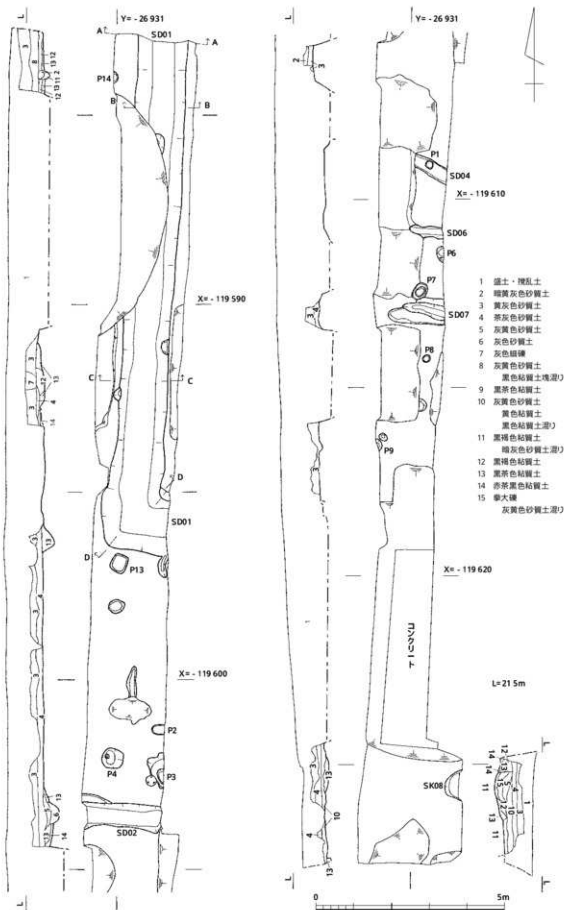
第3図 北調査区平安時代以降の遺構・土層図 (1/100)
