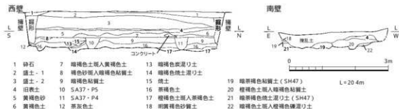
第7図 南調査区土層図(1/80)
