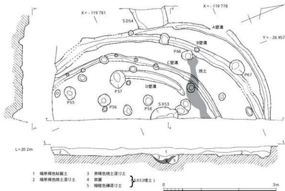
第12図 竪穴住居S H47実測図(1/50)
