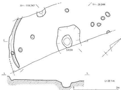
第13図 竪穴住居S H48実測図(1/50)
