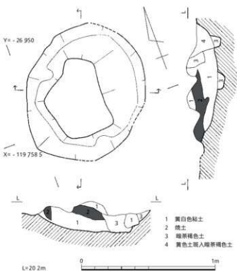
第9図 カマド S X 42実測図 (1/20)
