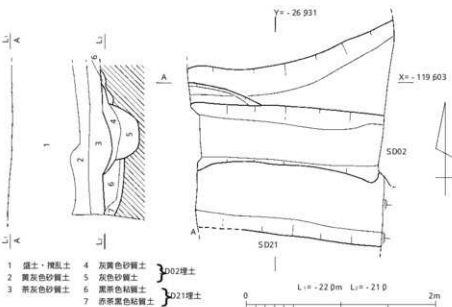
第 6 図 溝 S D02・21実測図 (1/40)
