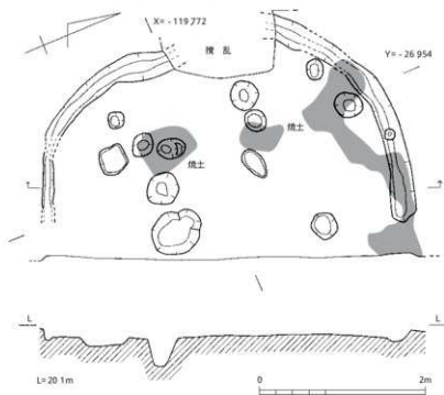
第14図 竪穴住居S H52実測図(1/50)
