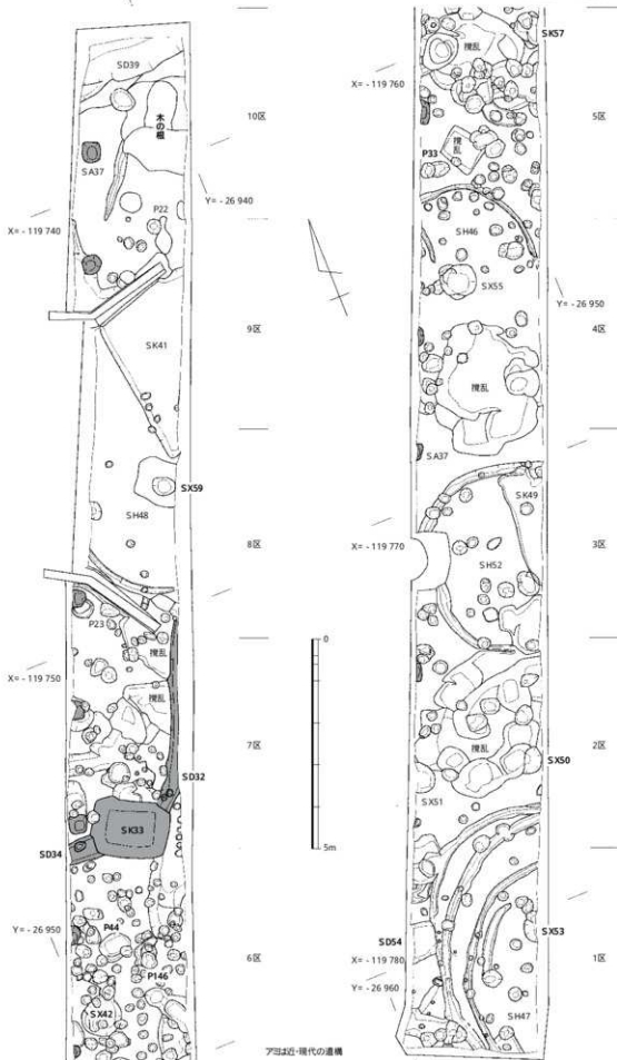
第8図 南調査区検出遺構図(1/100)
