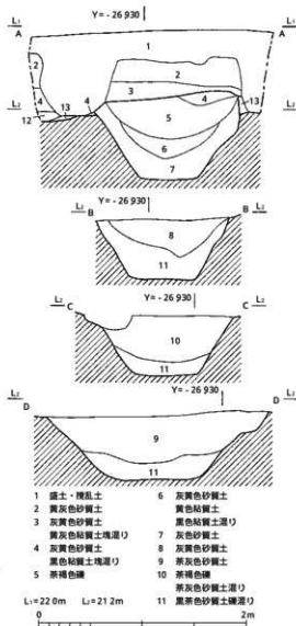
第4図 堀 S D01土層図 (1/40)
