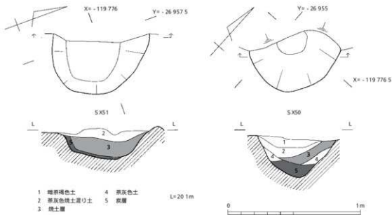
第15図 炉跡S X50・51実測図(1/20)
