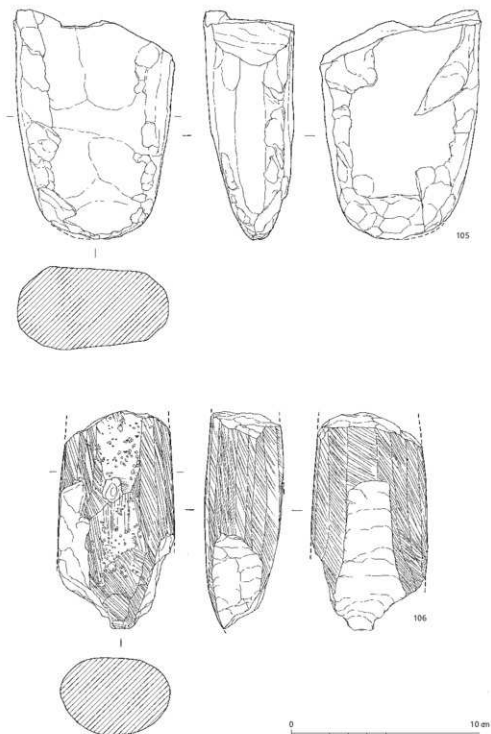
第23図 南調査区出土石器実測図 - 2 (1/2)
