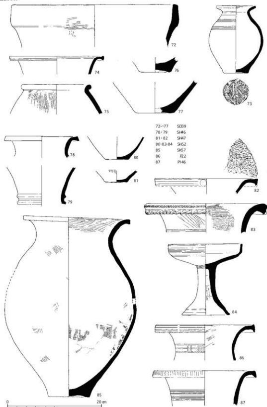
第21図 南調査区出土弥生土器実測図(1/4)
