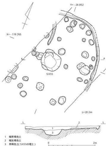
第11図 竪穴住居S H46実測図(1/50)
