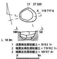
第 13 図 土坑 S K 13 実測図 (1.50)
