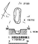
第10図 土坑SK 10実測図 (150)
