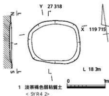
第 12 図 土坑 S K 08 実測図 (1.50)
