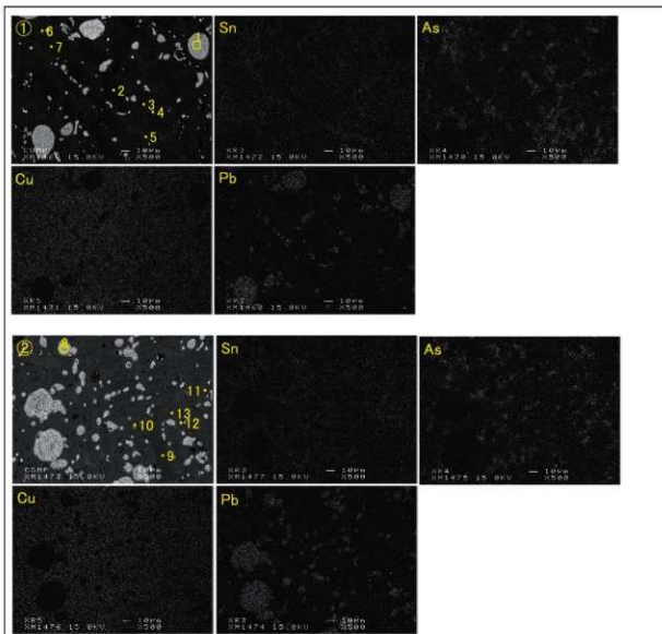
青銅部分の反射電子像(COMP)・特性X線像
