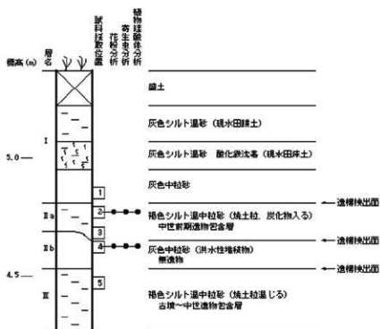
図1 D-15東壁の模式状況 凡例 ■ 酸化鉄 ▨ シルト
