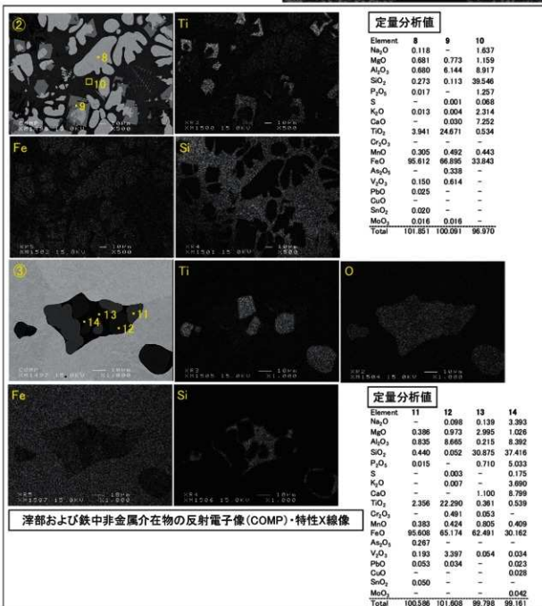
Photo. 13 椀形鍛冶滓 (鍛造品付) の顕微鏡組織・EPMA調査
