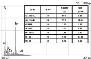
図2 試料2の成分分析(蛍光X線分析装置による)
