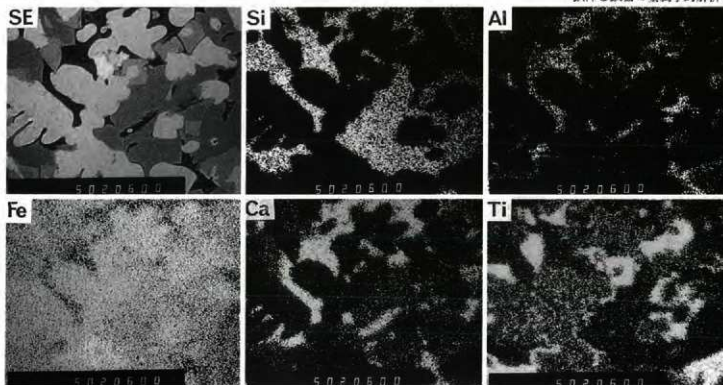
1 ③鉄滓の元素分布 (EPMA)
