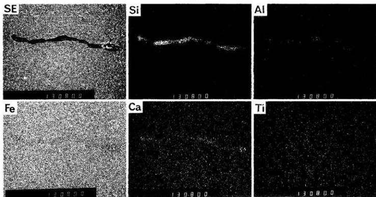
1 ⑬試料に存在する介在物の元素分布 (EPMA)
