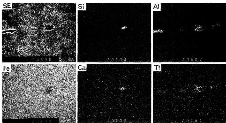
2 ②試料中在物の元素分布 (EPMA)
