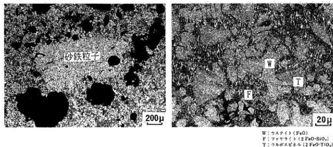
2 ⑬鉄滓の組織
