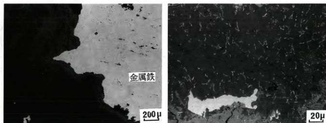
2 ⑬試料の断面組織
