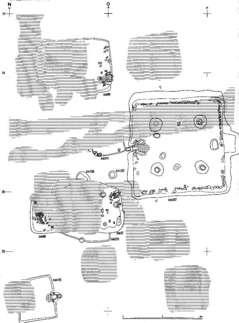
古代遺構図30 (1:120)
