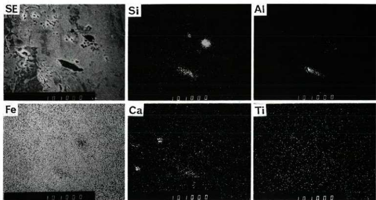
1 ⑧試料中に存在する介在物の元素分布 (EPMA)
