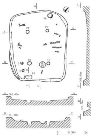
図9 SB1実測図
