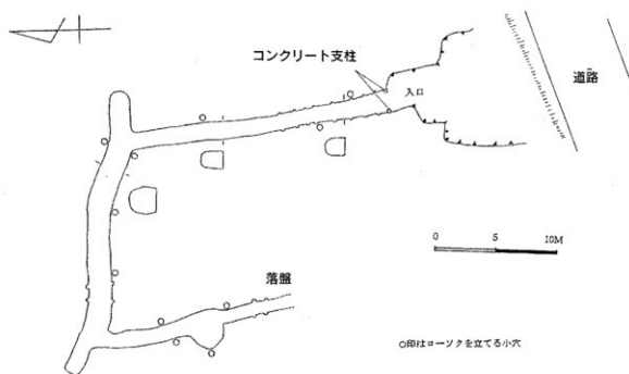
第11図 小波津の陣地壕平面遺構図 西原町教育委員会提供
