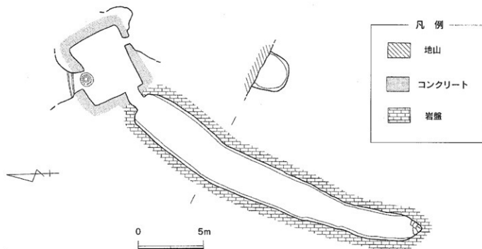
第12図 海軍砲台跡平面遺構略図
