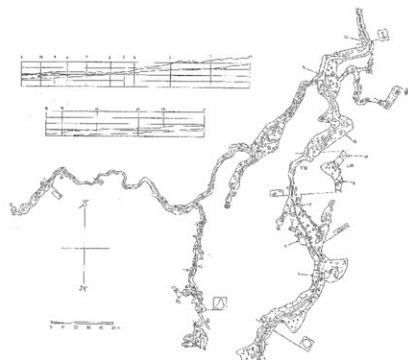
第24図 シムクガマ平面図 『沖縄県洞穴実態調査報告II』沖縄県教育委員会 1979年より
