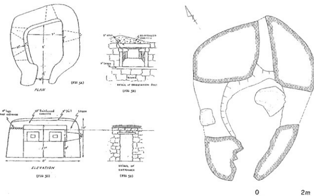
第20図 トーチカ平面図及び立面図 [Intelligence Monograph, RESTRICTED RYUKYU CAMPAIGN G-2 TENTH ARMY, 15 JULY 1945] より
