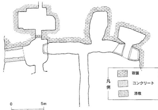
第7図 海軍砲台跡平面遺構略図
