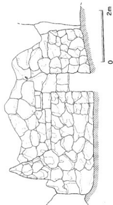
第22図 大城の銃眼平面図及び立面図
