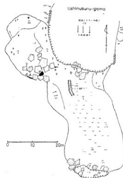
第16図 ウシヌスルガマ平面図及び断面図 嘉手納町教育委員会提供
