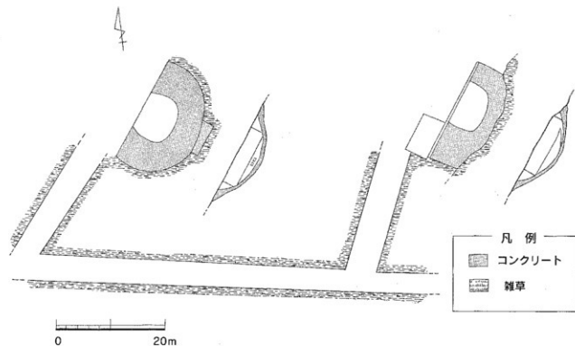
第25図 座喜味の掩体壕群平面図及び立面図
