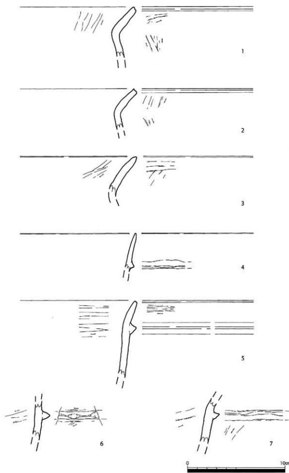
第17図 出土遺物実測図①(S=1/2)
