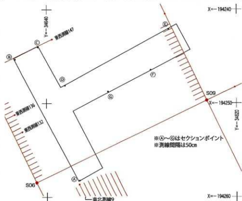
第5図 トレンチ位置と地中レーダ調査測線(S=1/200)
