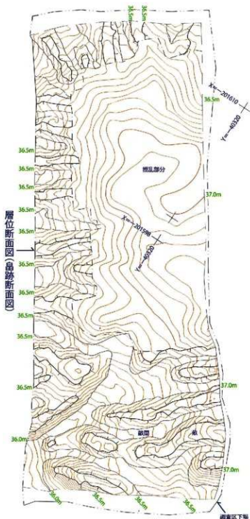
第24図 畝跡コンタ図(S=1/200)
