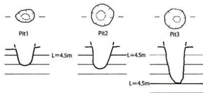
第14図 ビット平・断面図(S=1/20)
