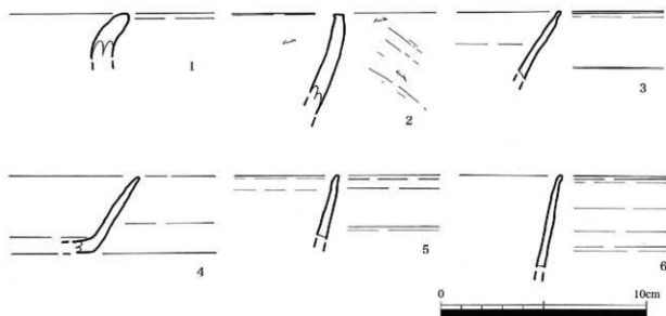
図10 出土遺物実測図 (S=1/2)
