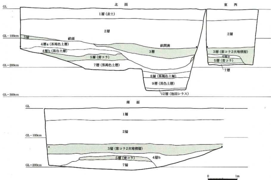
図13 大園原遺跡 1トレンチ層位断面図 (S=1/40)
