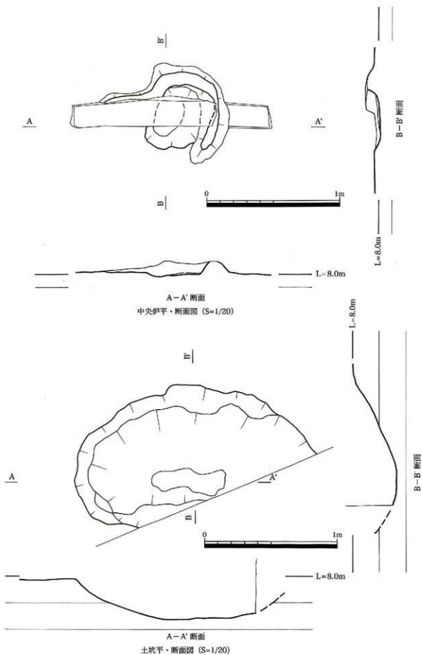
图9 中央炉及び土坑平・断面图 (S=1/20)
