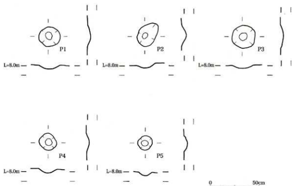
図8 ビット平・断面図 (S=1/20)
