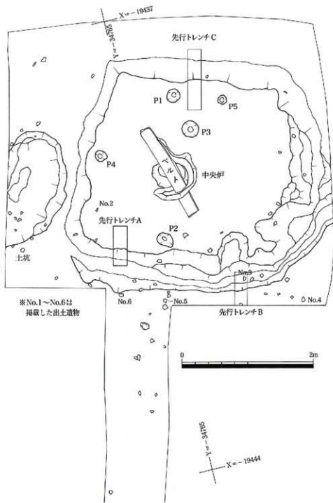
図5 遺構配置図 (S=1/40)
