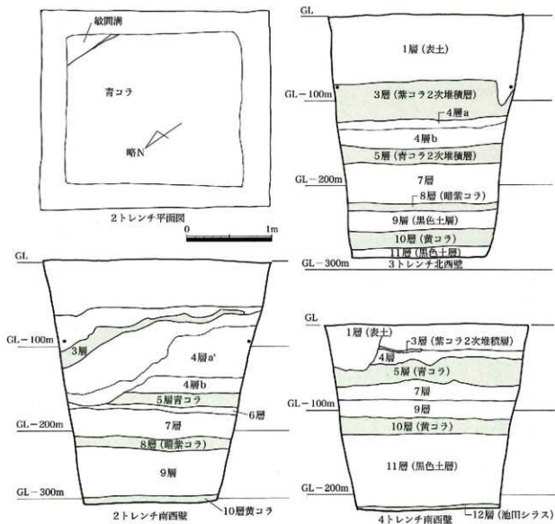
図14 2, 3, 4トレンチ 層位断面図 (S=1/40)
