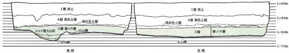
図6 層位断面図 (S=1/40)
