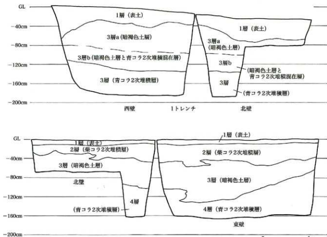
図17 山王遺跡層位断面図 (S=1/40)
