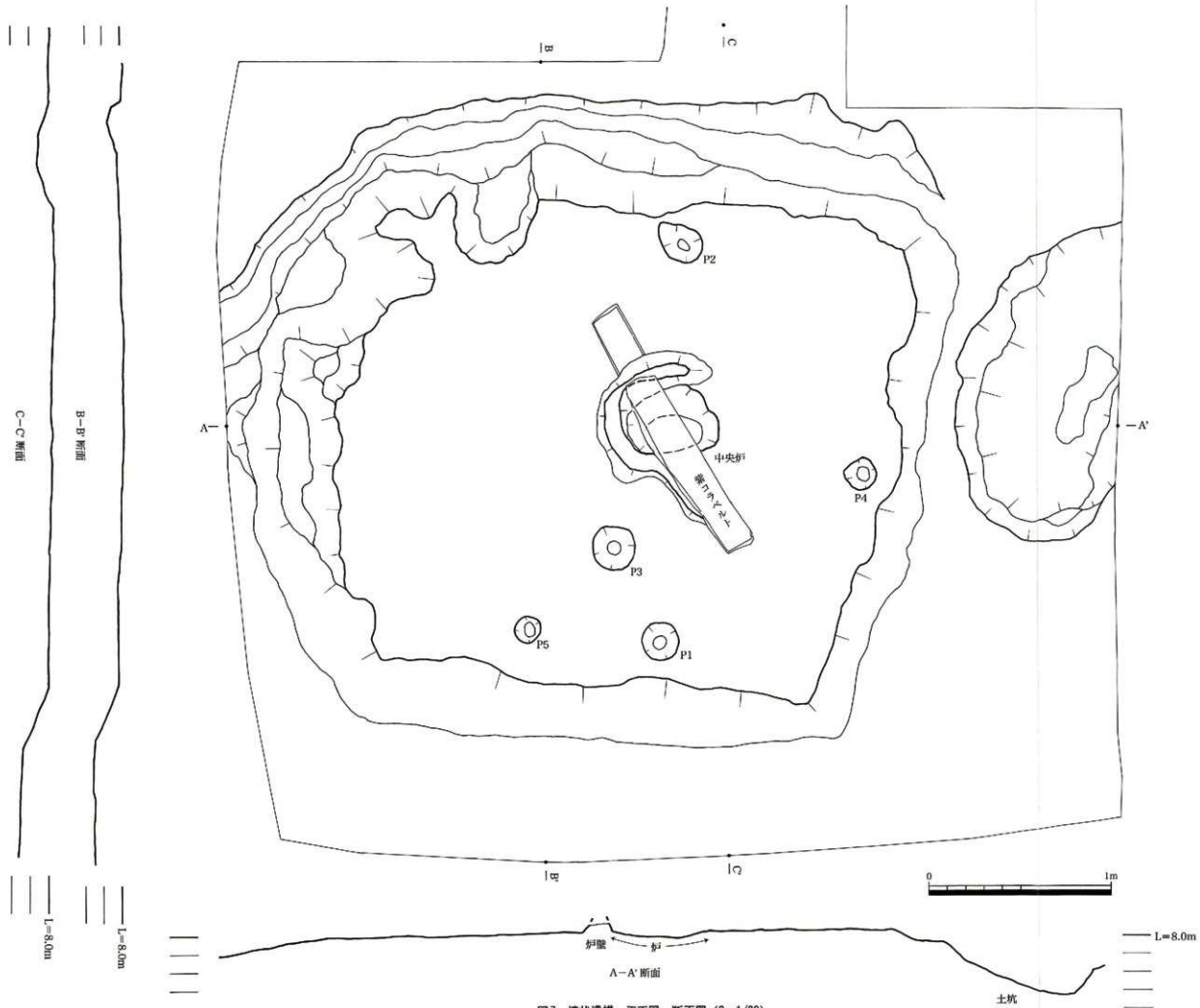
図7 塚状遺構 平面図・断面図 (S=1/20)
