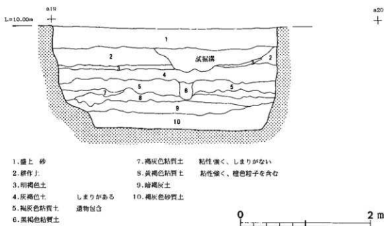
第19図 a19～a20セクション図
