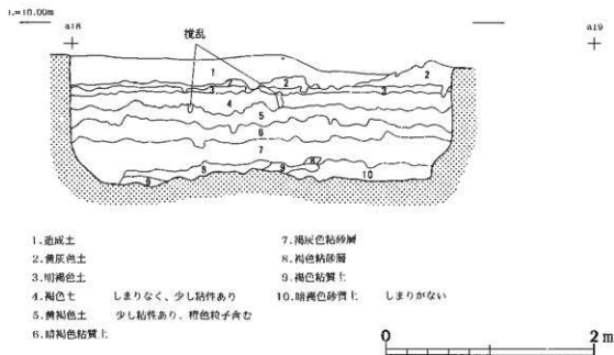
第17図 a16~a19セクション図
