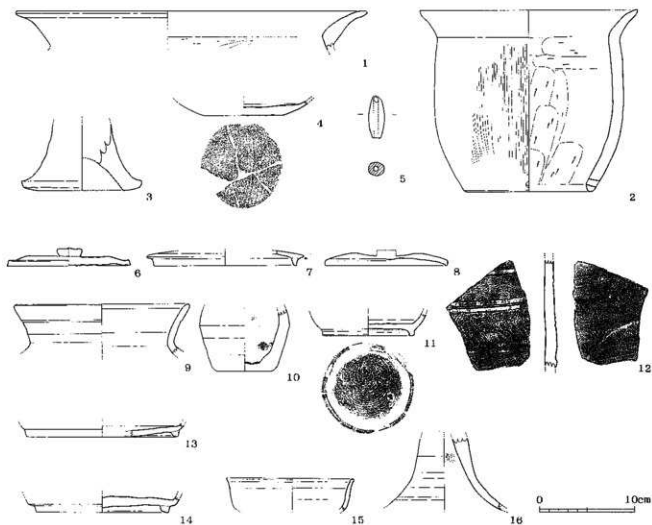
第10図 SD01出土遺物実測図
