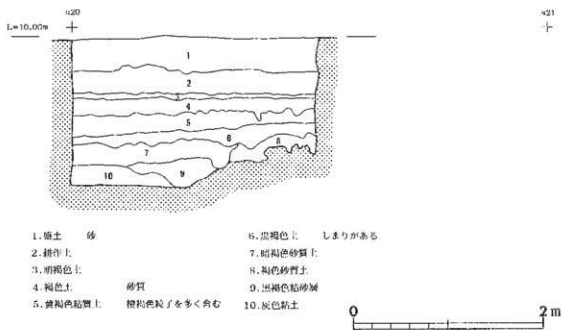
第21図 a20~a21セクション図
