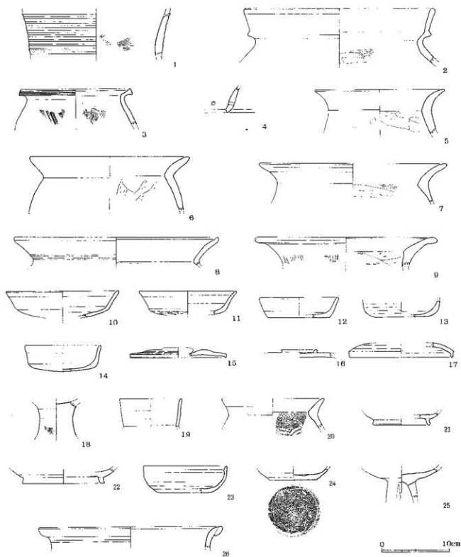
第13図 11~13G r 出土遺物実測図
