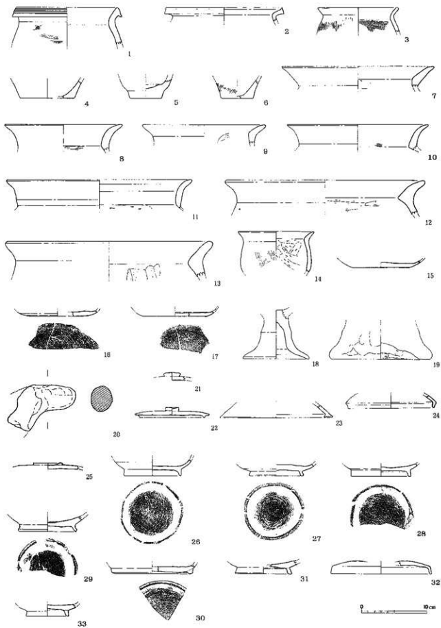
第14图 14~16Gr出土文物实测图(1)
