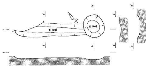
第5図 遺構実測図
