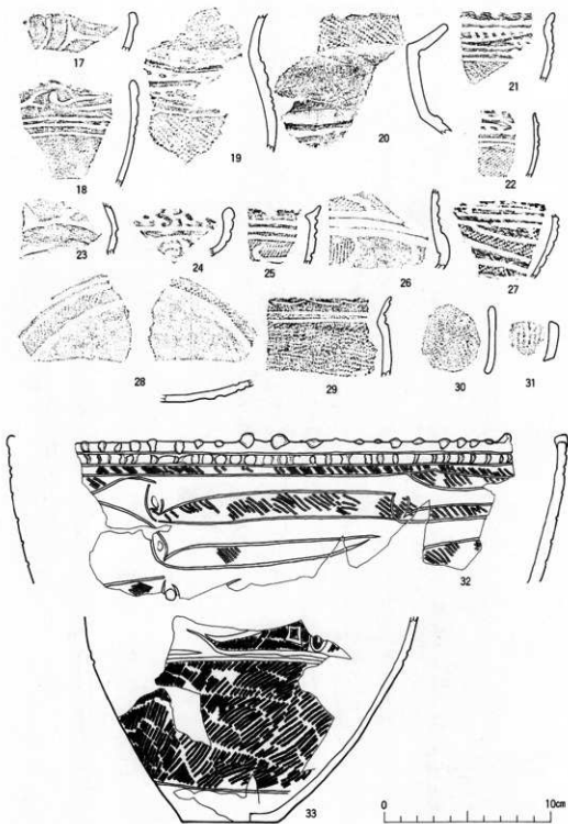
第5図 Dh29・30 出土土器・土製品
