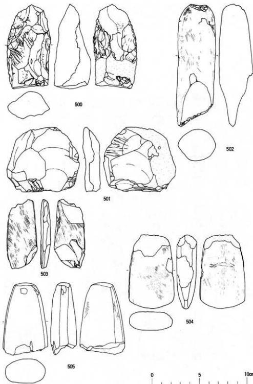
第35圖 Eh40・Fa41 出土石器
