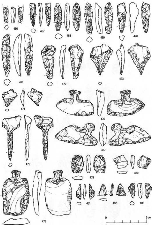
第33图 Eh40·Fa41 出土石器
