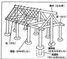
ほったてばしら 掘立柱建物の構造
