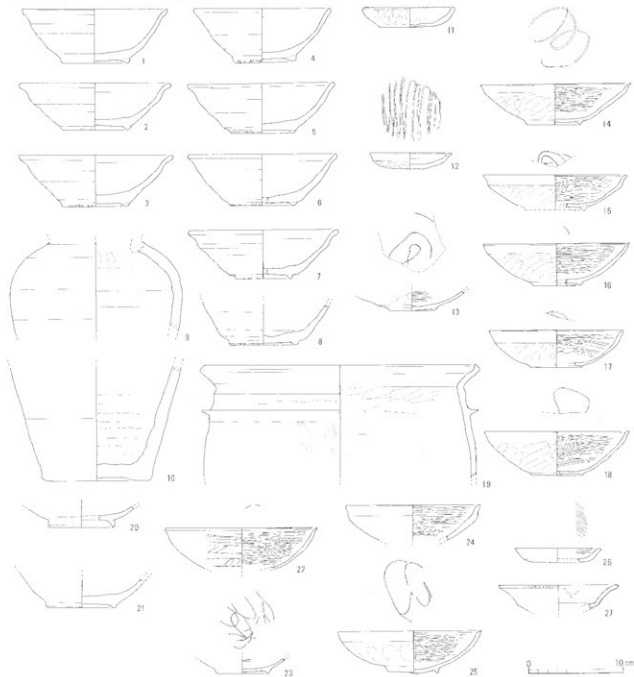
第26図 出土遺物実測図 (1) SK37・SD30 (S=1:4)
