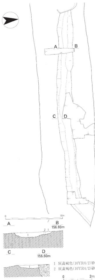
第23図 SD 11平面図 (S = 1 : 200) 及び土層断面図 (S = 1 : 80)
