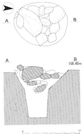
第21図 SK 18出土状況図 (S = 1 : 20)
