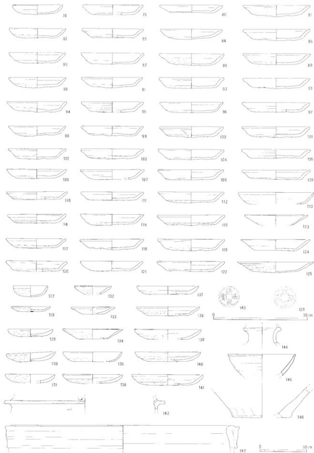
第28图 出土物实测图(3) SK3・4 (S=1:4)
