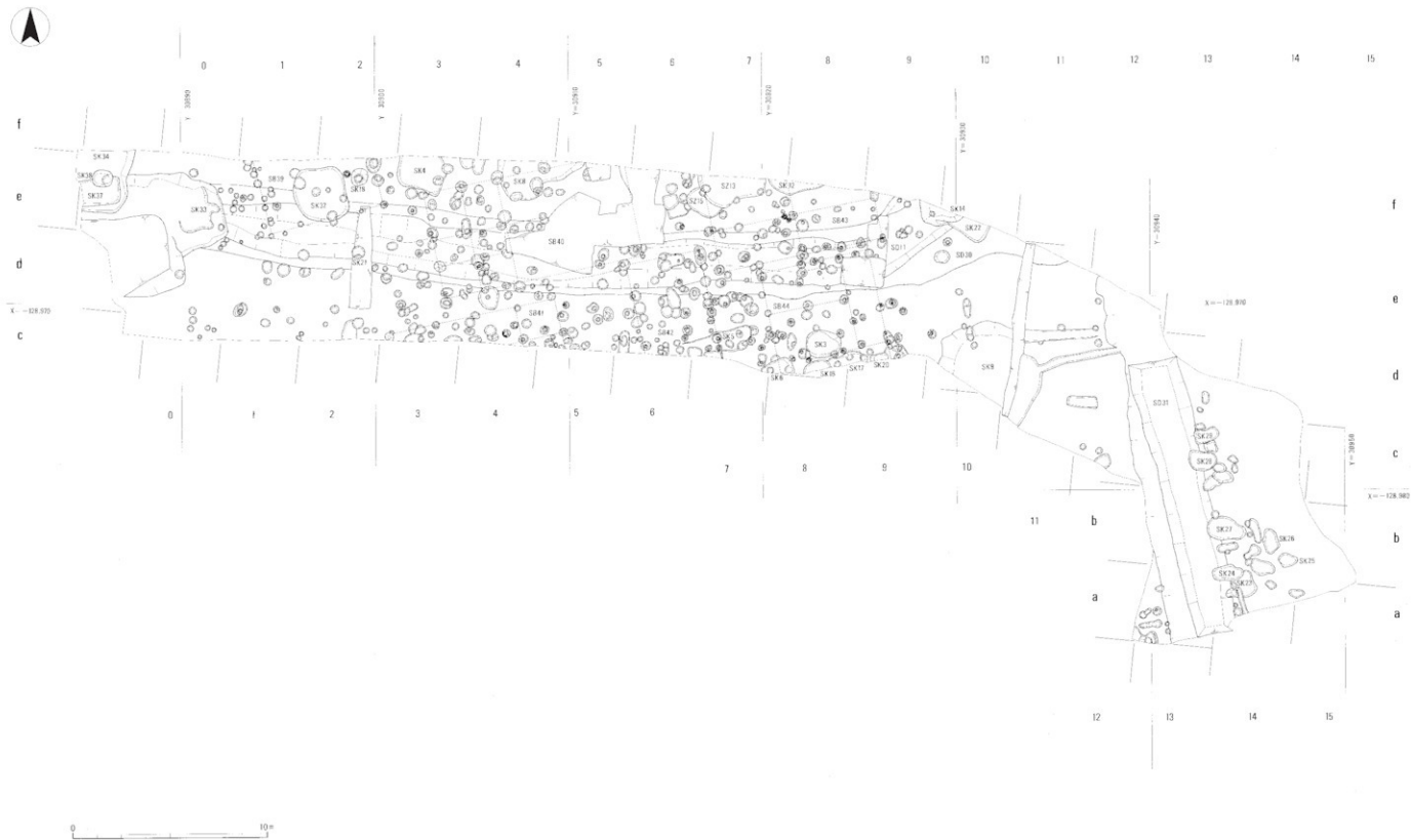
第7図 第2面遺構平面図 (S = 1 : 200)
