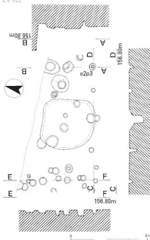
第10図 SB39平面図及び断面図（S=1:100）
