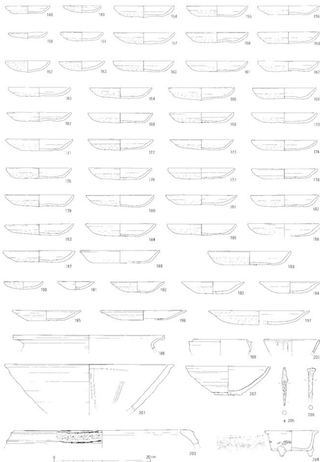
第29図 出土遺物実測図(4) SK8 (S=1:4)
