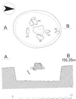
第22図 SK 21出土状況図 (S = 1 : 20)
