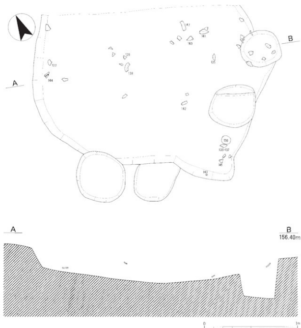
第15図 SK 4出土状況図 (S = 1 : 20)
