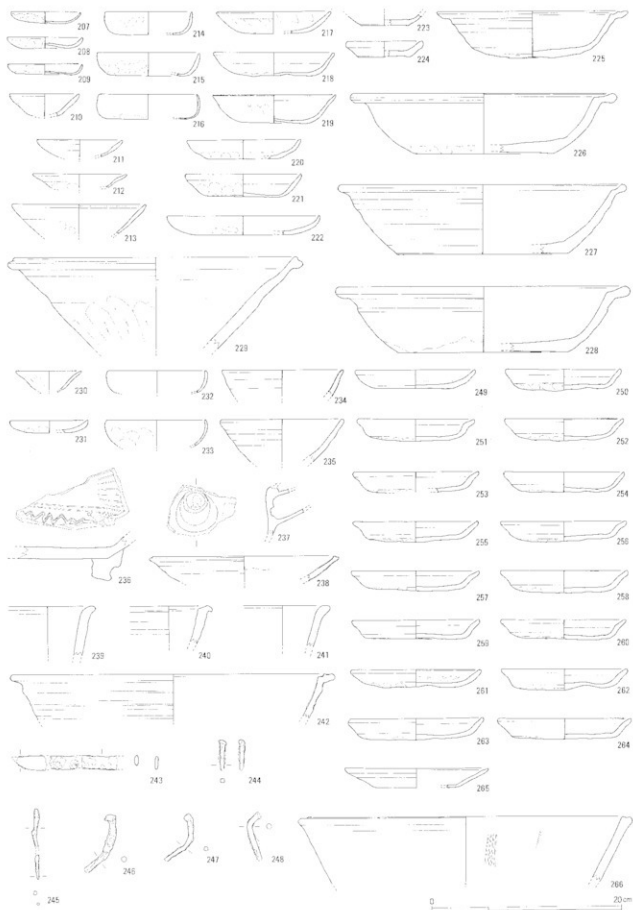
第30图 出土遺物実測図(5) SK9・14・22 (S=1:4)
