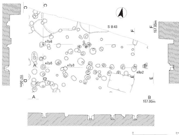
第13図 SB43平面図及び断面図（S = 1 : 100）
