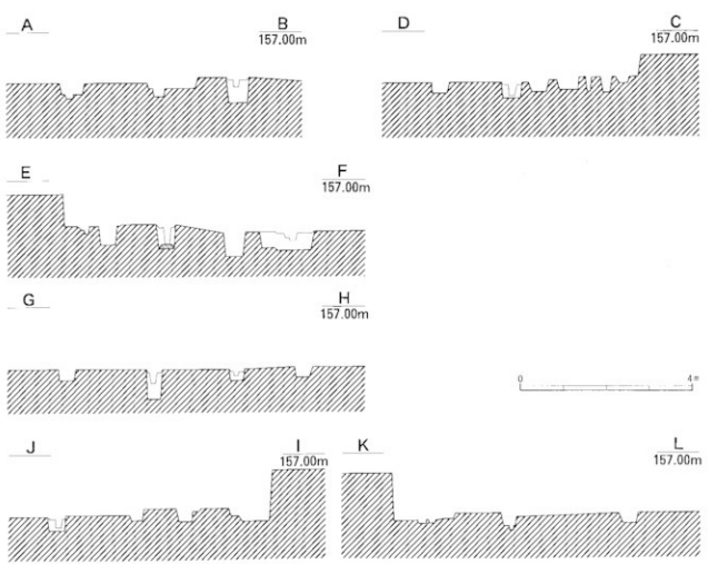
第12図 SB42・44平面図及び断面図 (S = 1 : 100)
