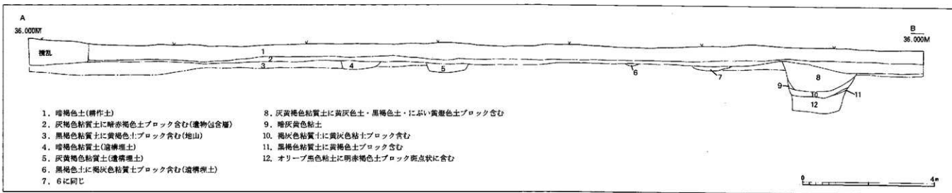
第5図 調査区(B区)西壁土層断面図 (1:80)
