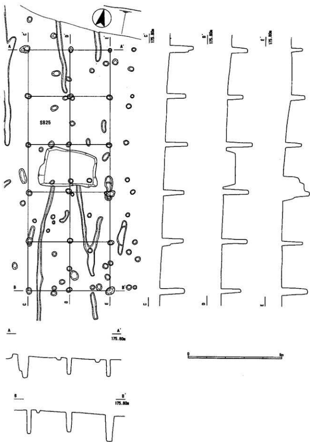
第9図 西山遺跡 遺構実測図4 1:100 SB25
