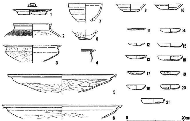
第8図 野田遺跡出土遺物 1 : 4
