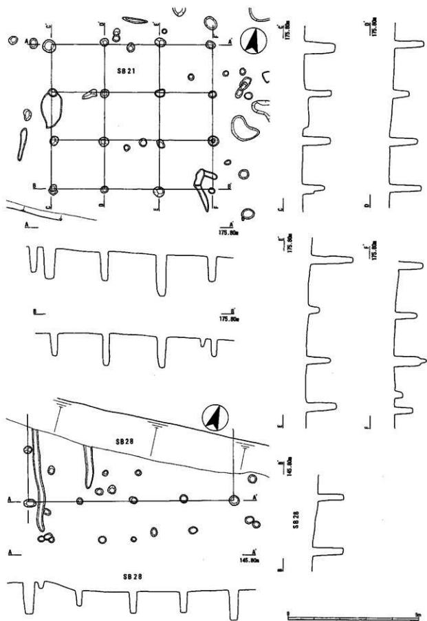
第6圖 西山遺跡 遺構実測圖 1 1 : 100 SB21・28
