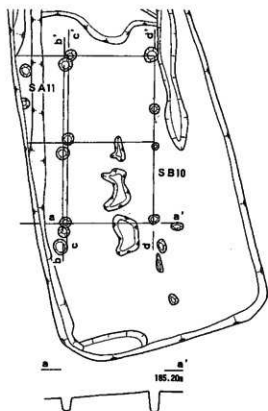
第16图 中出向遺跡SB10・SA11遺構実測図 1:100
