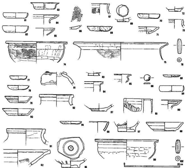
第9図 出土遺物実測図2 1:4
