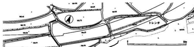
第21図 間所遺跡 トレンチ設定図 1:1,000
