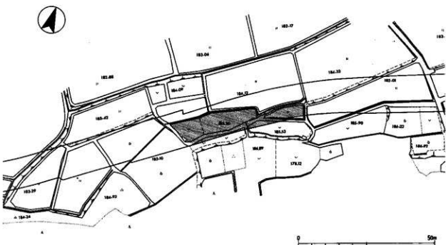
第14図 中出向遺跡 調査区位置図 1:1,000
