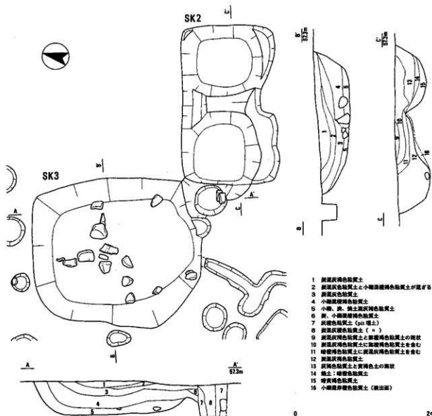
第6図 SZ14石列、SK23、SK2・3平面図・断面図・側面図 1:40
