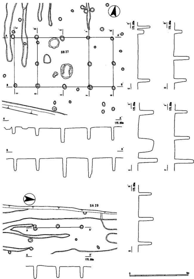
第11圖 西山遺跡 遺構実測圖6 1:100 SB27-SA29
