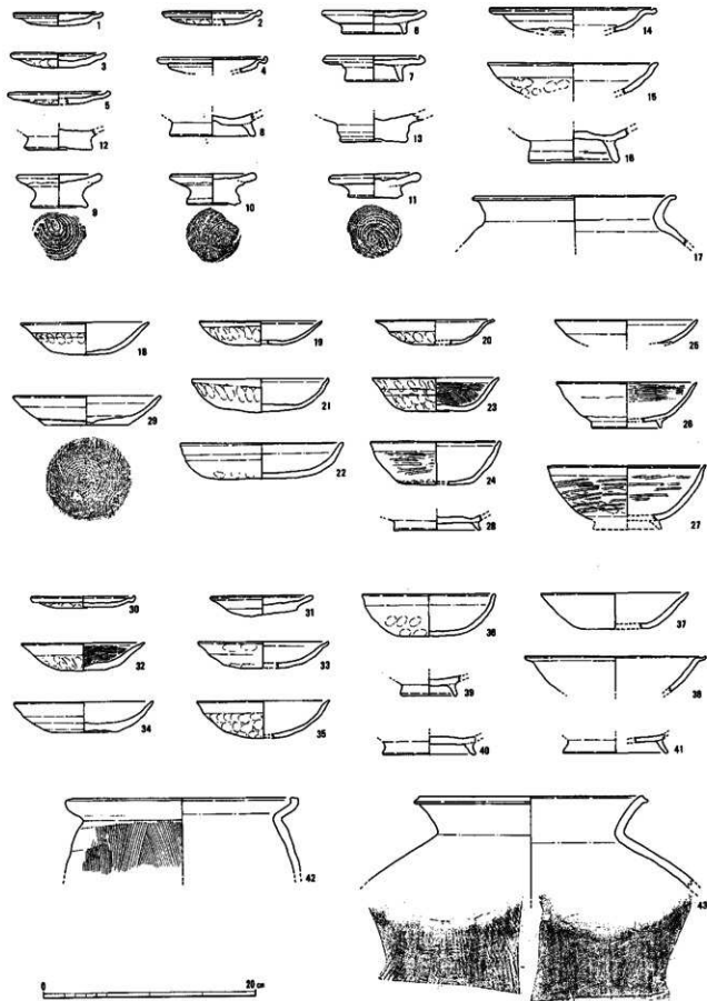
第12圖 西山遺跡 遺物実測図 1:4
