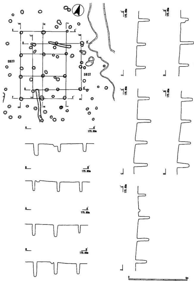
第7图 西山遺跡 遺構実測図2 1:100 SB22-23
