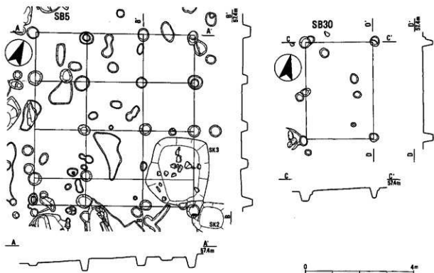
第5図 SB5、SB30平面図・断面図 1:100
