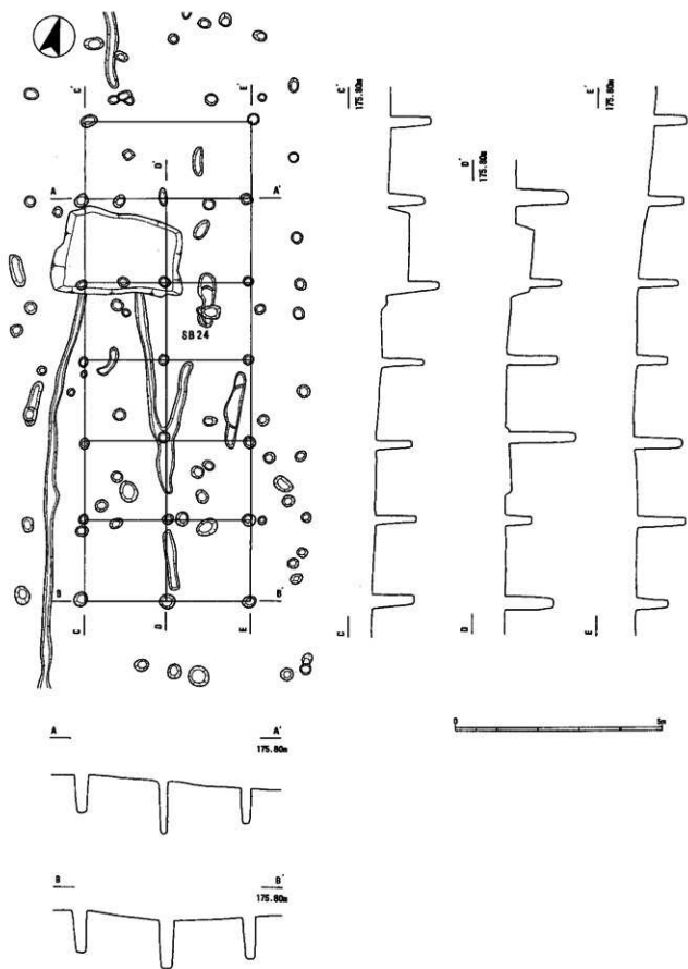
第8圖 西山遺跡 遺構実測図3 1:100 SB24
