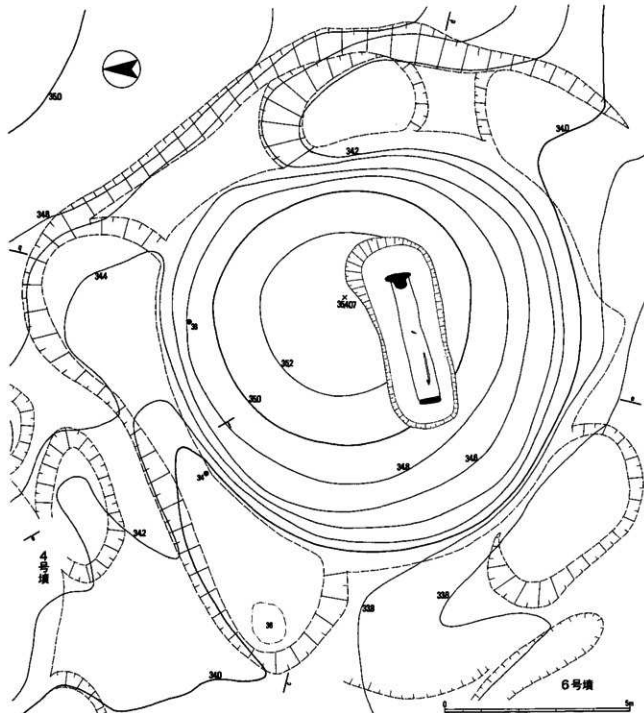
fig. 16 2号墳平面図 (1:100)
