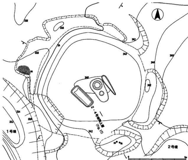
fig. 30 4号墳平面図(1:100)
