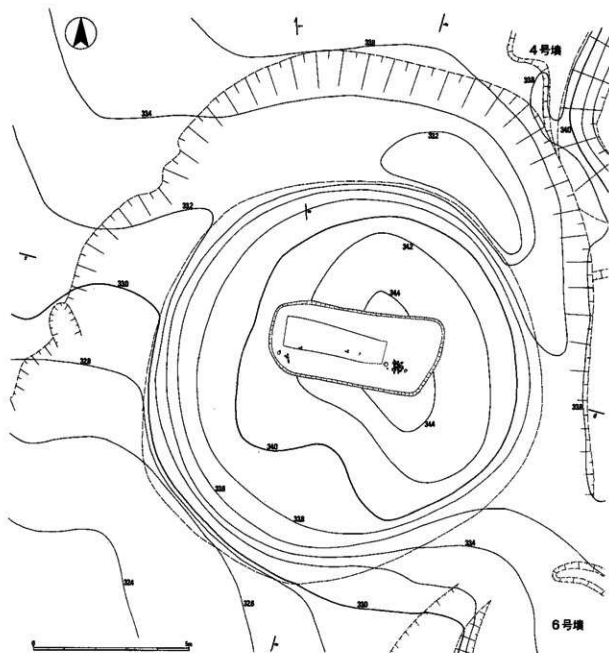
fig. 8 1号墳平面図 (1 : 120)
