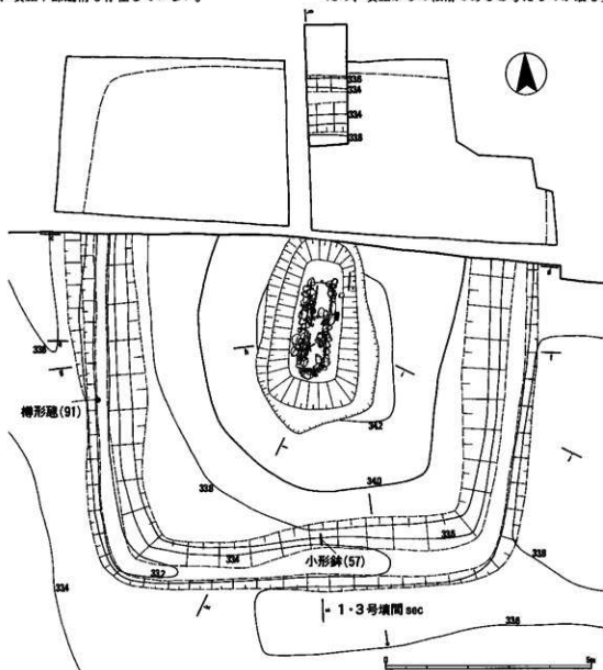
fig. 21 3号墳平面図 (1:100)
