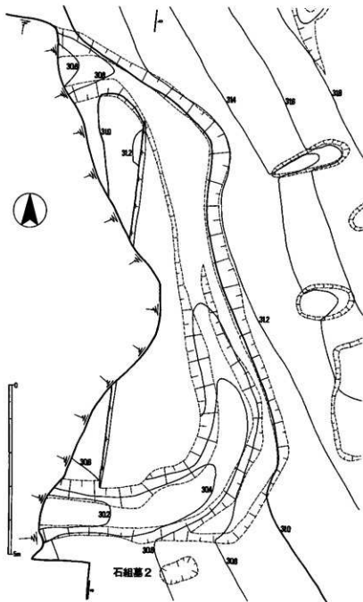
fig. 41 7号墳平面図 (1:100)
