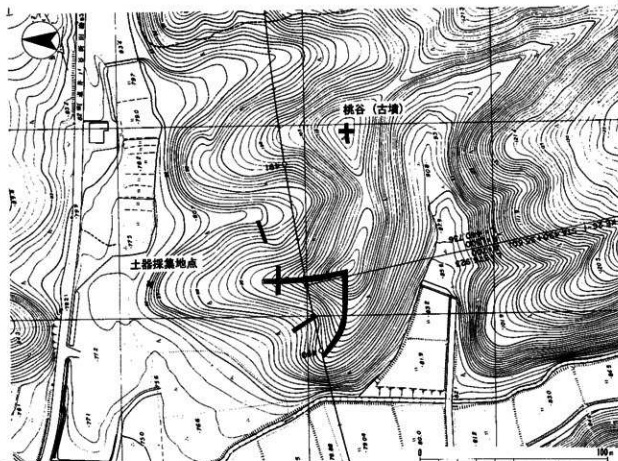
第21図 発掘区位置図(1:2,000)
