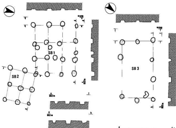
第12图 SB1・SB2・SB3実測图(1:100)
