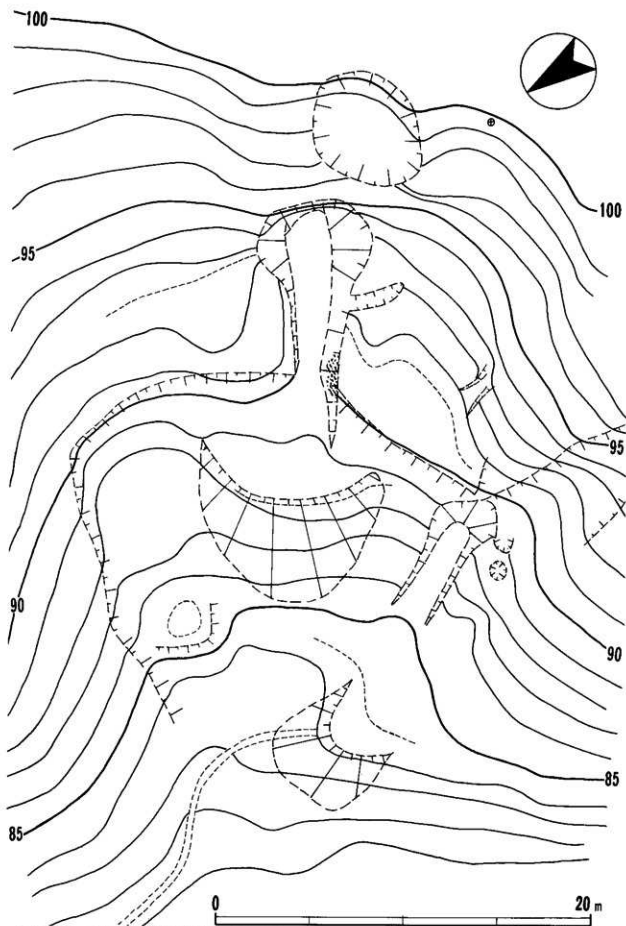
第4图 1·2号坑I附近地形测量图(1:200)
