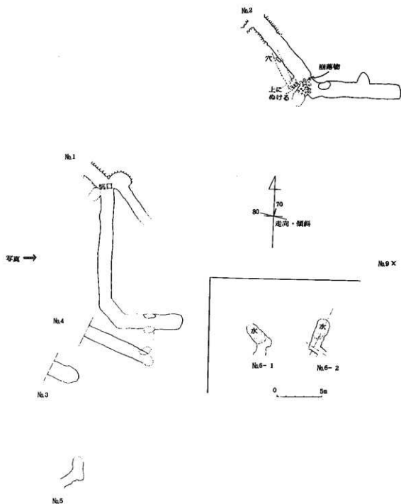
図4 佐奈鉱山跡分布図 (1989年7月21日調査)
