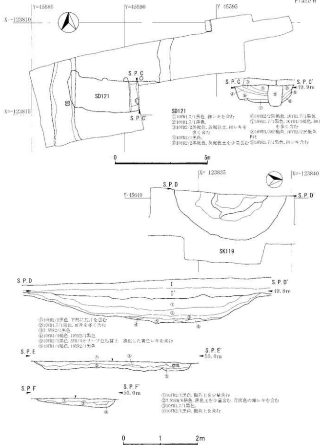
6AHD-D-2区平面図(1:100) 溝SD121断面図(1:50) 土坑SK119平面図(1:100) 土坑SK119-SK124断面図(1:50)
