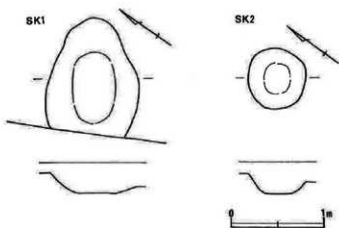
図6 遺構 (1/40)
