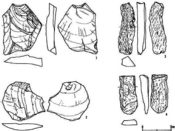
図7 石器実測図 (1/2)
