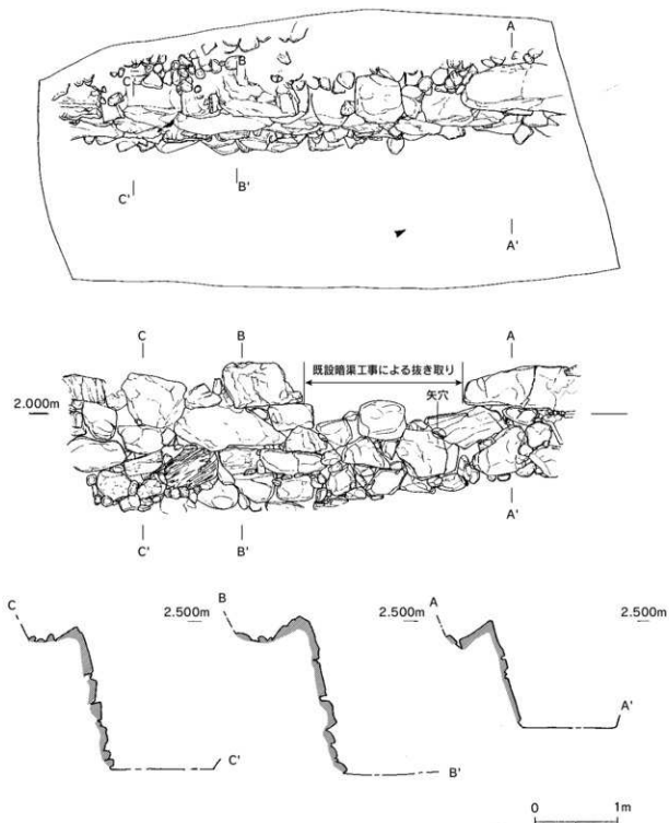
第14図 平面図・立面図・断面図 (S=1/50)
