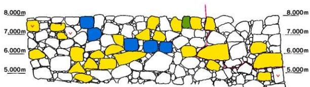
第21図 N面 (S=1/100)
