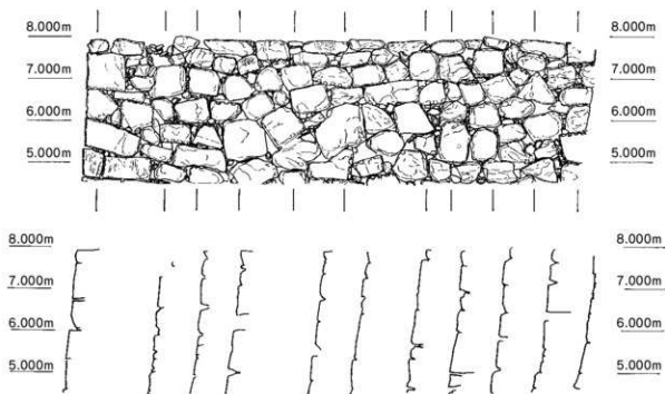
第16図 o面 (S=1/100)
