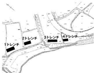
第10図 トレンチ配置位置図 (S=1/15,000)
