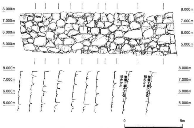
第17図 N面 (S=1/100)
