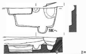
III-386 112号住居址、イ号溝址実測図
