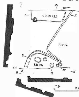
III-424 185号・189号(上)住居址実測図
