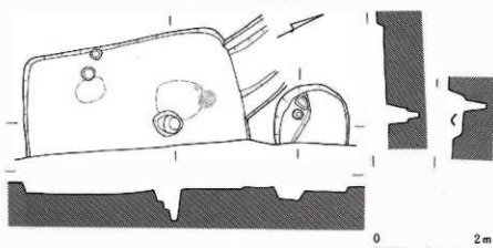
III-247 57号住居址実測図
