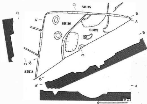
III-182 128号住居址実測図
