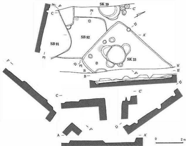
III-273 92号・93号・98号住居址，土構33・39実測図
