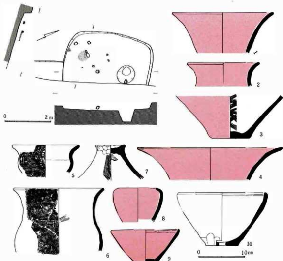
III-242 43号住居址実測図・出土土器
