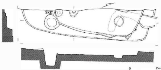
III-257 71号・72号住居址実測図
