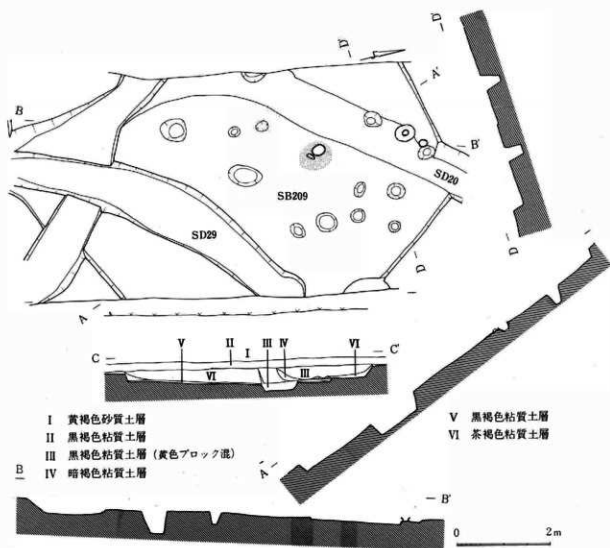
III-187 209号住居址, 29号溝址実測図
