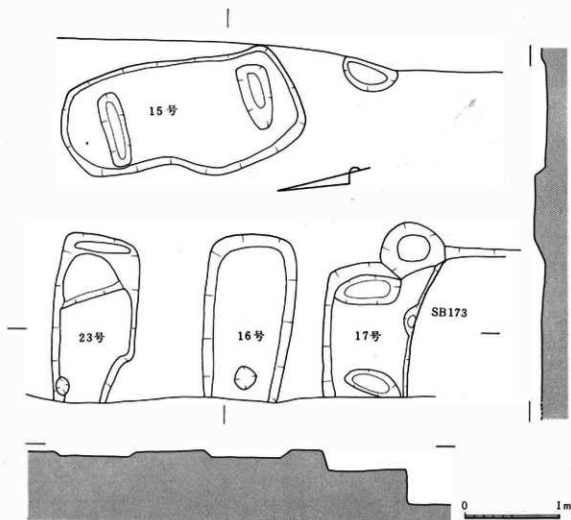
III-138 第V墓塚群実測図
