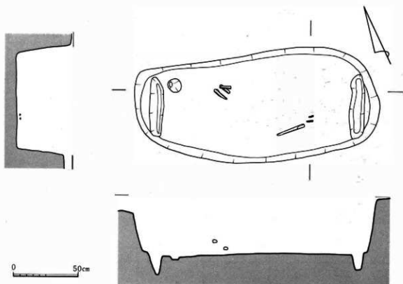
III-130 14号木棺墓実測図
