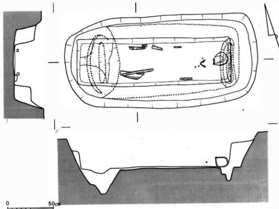
III-132 22号木棺墓実測図
