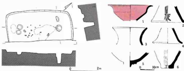
III-227 31号住居址実測図・出土土器
