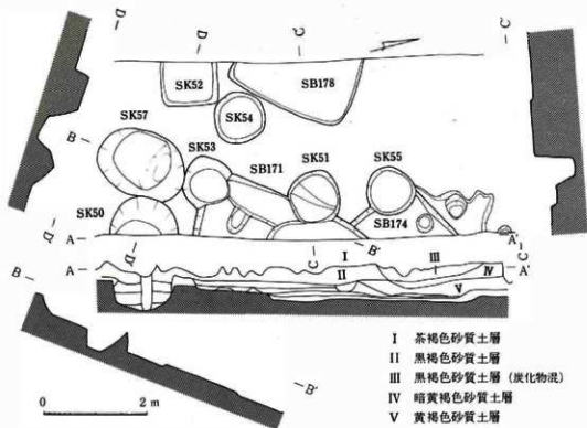
III-185 178号・171号・174号住居址、土壌50-55実測図
