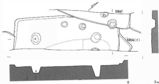
III-228 34号(ロ)・47号住居址実測図
