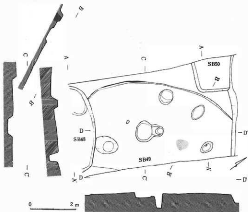
III-179 49号住居址実測図
