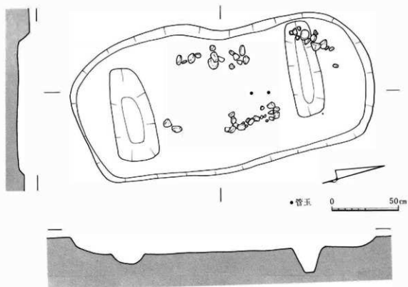
III-139 15号木棺墓実測図
