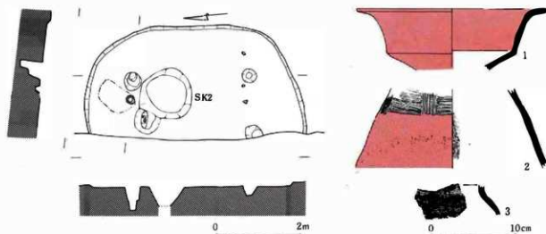
III-209 12号住居址，土壙2実測図，12号住居址出土土器
