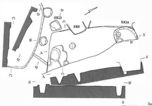
III-218 21号住居址、土壇13・14実測図
