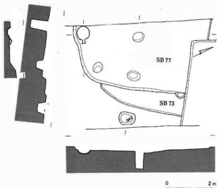
III-260 73号・77号住居址実測図
