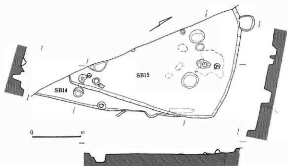
III-210 14号・15号住居址実測図
