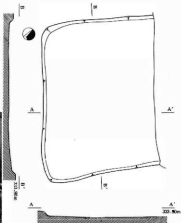
図17 10号住居址実測図(1:60)
