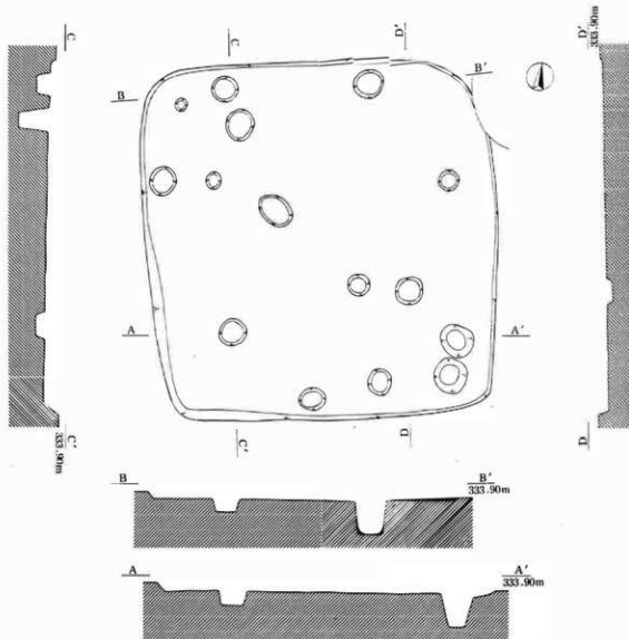
図5 1号住居址実測図
