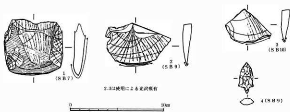
図23 出土石器実測図
