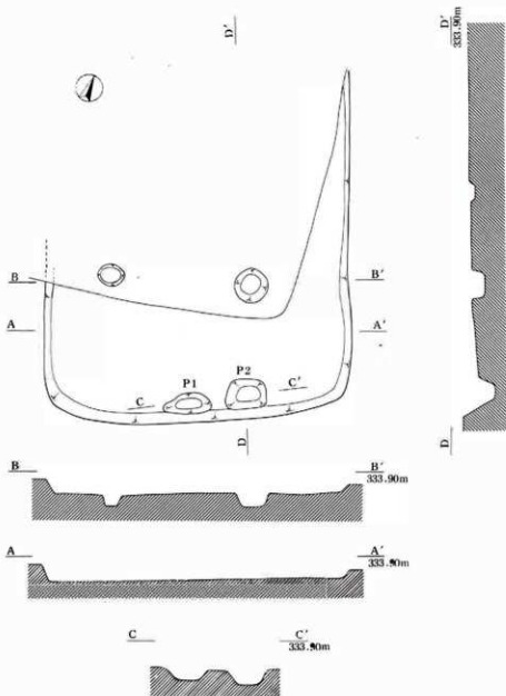
図7 2号住居址ならびに出土土器実測図
