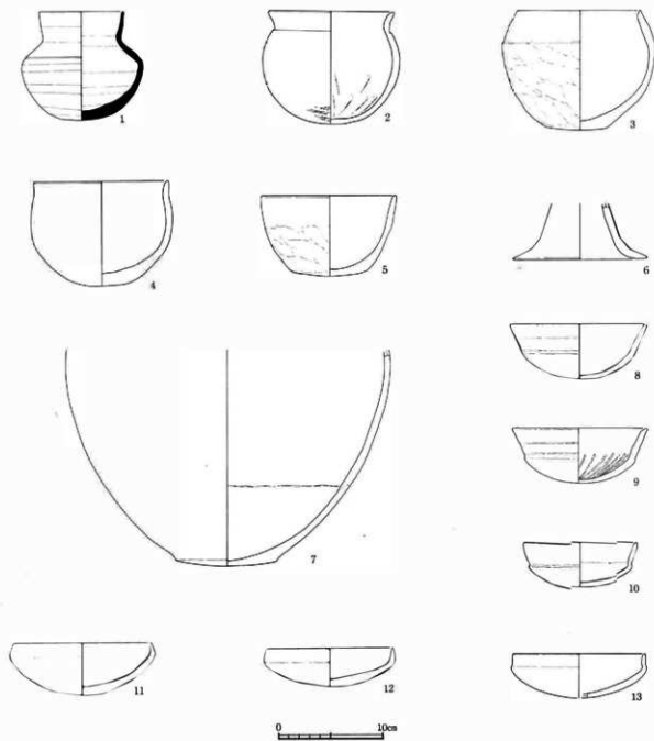
图6 1号住居址出土土器实测图
