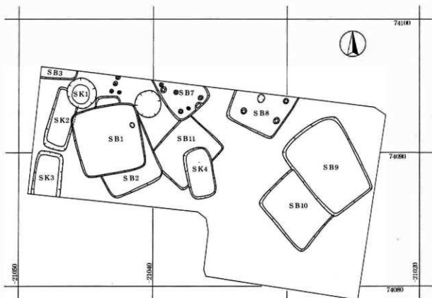
图4 调查区全测图 (1:200)
