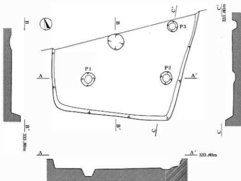
図13 8号住居址実測図(1:60)
