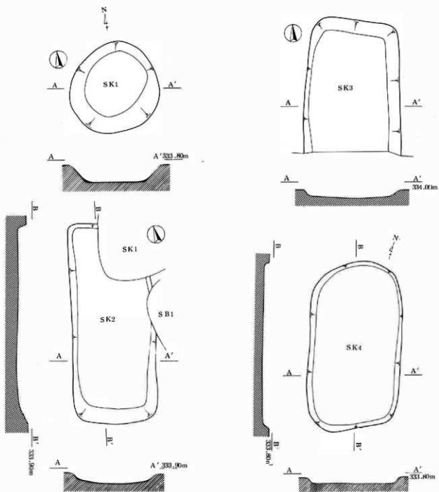
图20 1号~4号土坑实测图(1:60)
