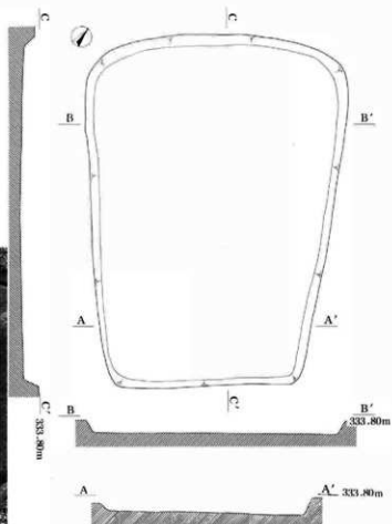
図15 9号住居址実測図(1:80)
