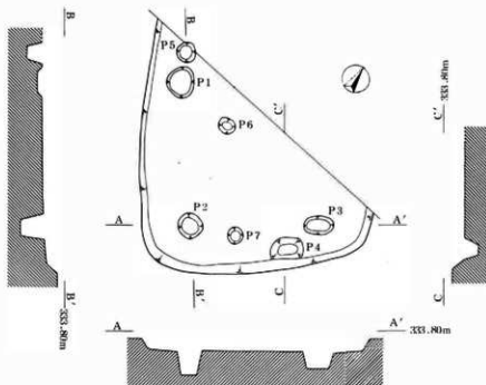
図11 7号住居址実測図(1:60)
