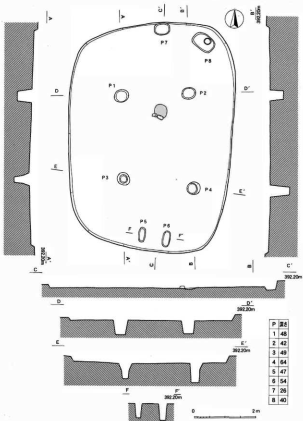
第60図 24号住居址実測図 (1 : 60)
