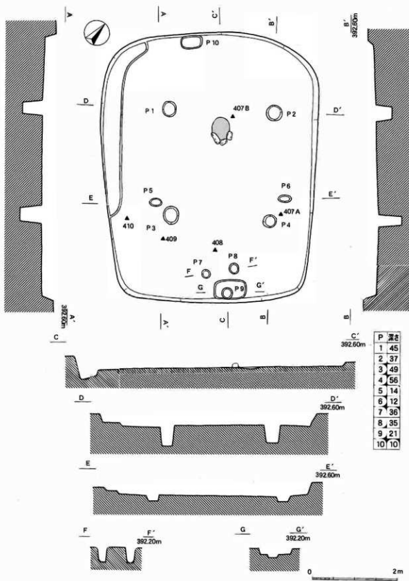
第44图 20号住居址实测图 (1:60)
