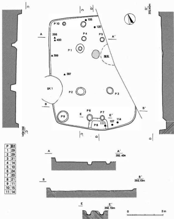
第28図 16号住居址実測図 (1:60)
