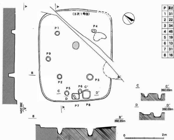
第24图 15号住居址实测图 (1:80)
