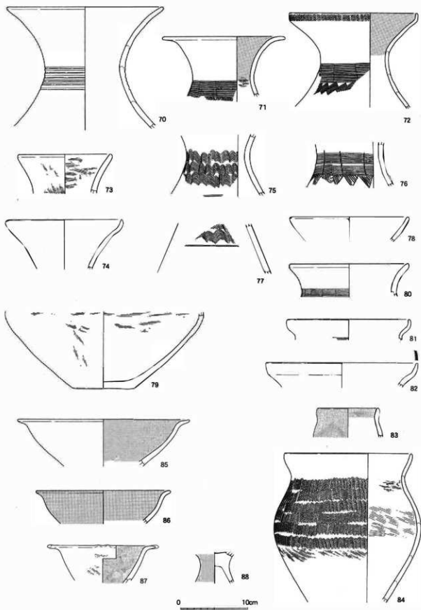
第19图 13号住居址出土土器实测图 (1:4)
