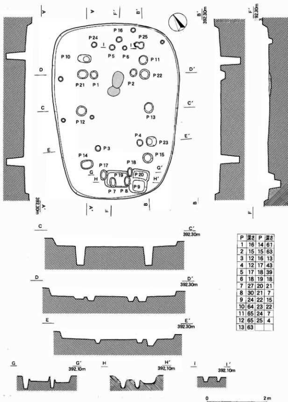
第31图 17号住居址実測図 (1:60)
