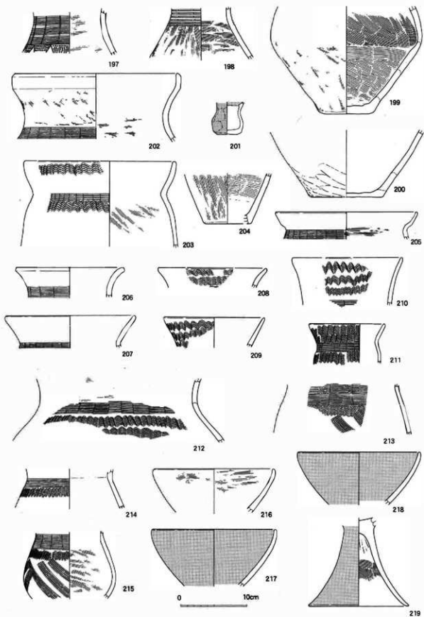
第52图 22号住居址出土土器实测图② (1:4)
