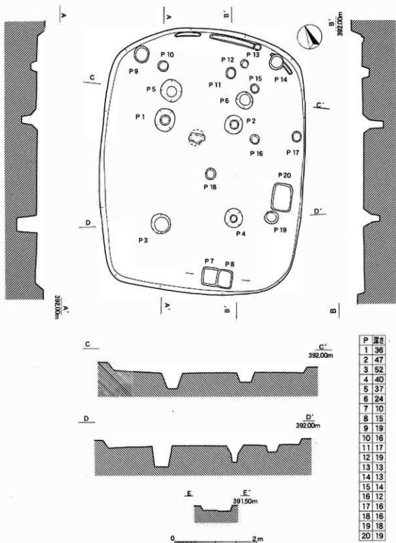
第18図 13住居址実測図 (1:60)
