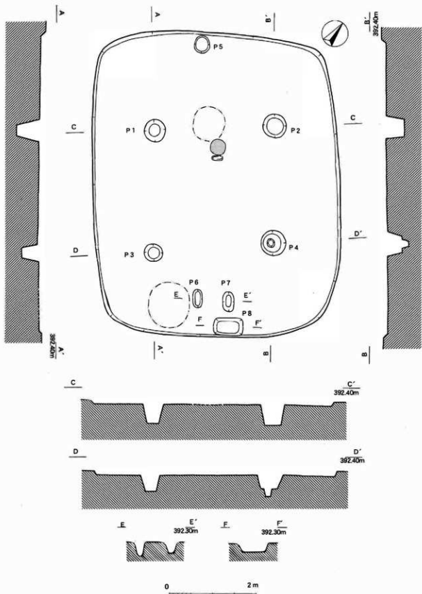
第76图 28号住居址实测图 (1 : 60)
