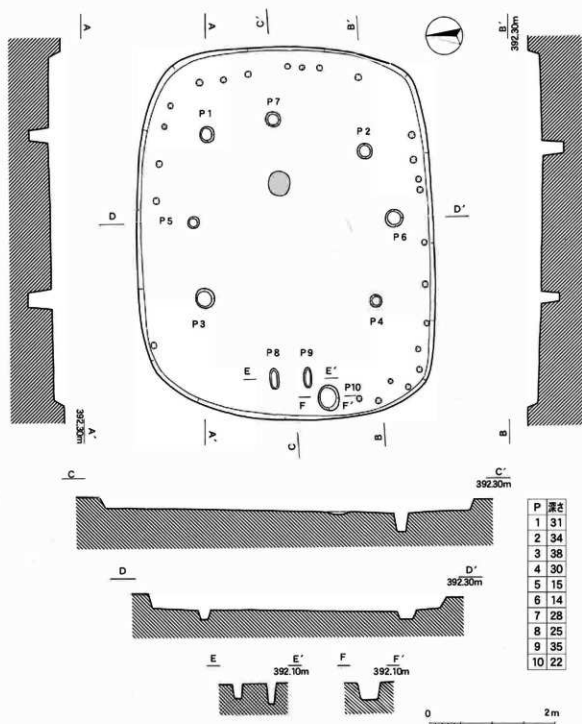
第55図 23号住居址実測図 (1:60)
