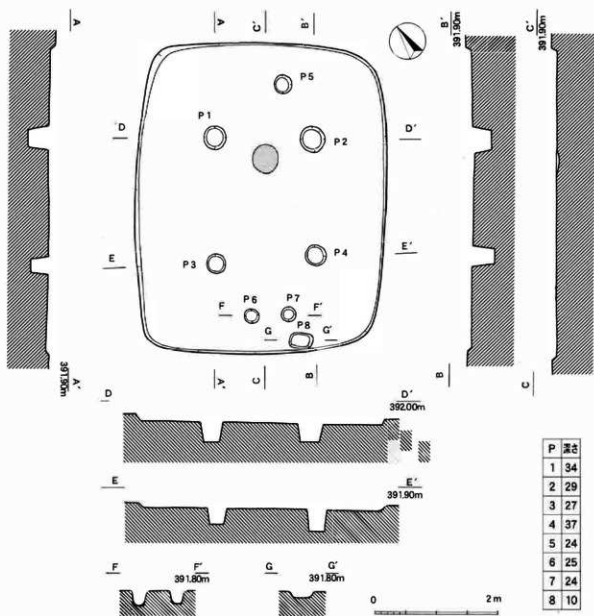
第71图 27号住居址実測図 (1:60)
