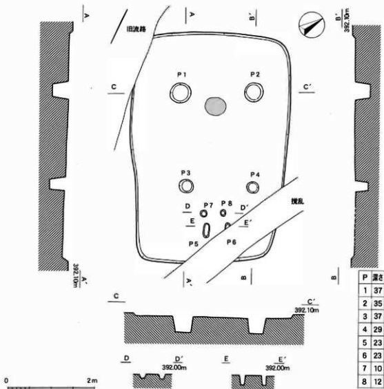
第67图 26号住居址实测图 (1:60)
