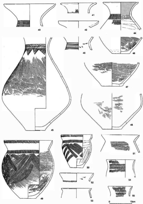
第14图 12号住居址出土土器実測図① (1:4)
