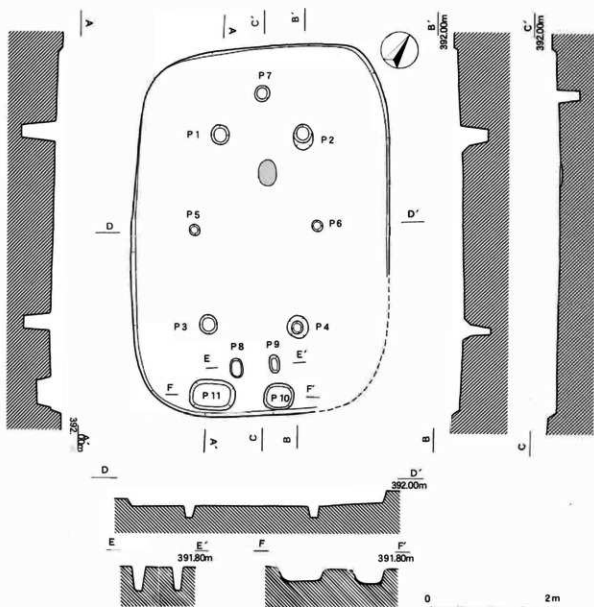
第63図 25号住居址実測図 (1 : 60)
