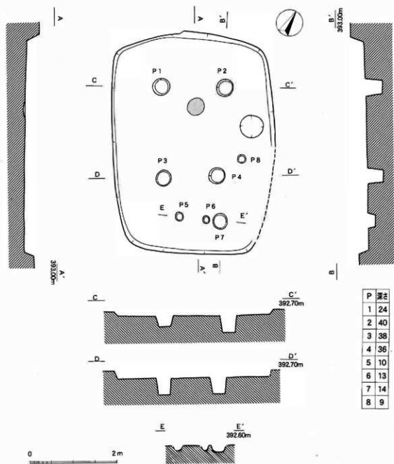
第37図 19号住居址実測図 (1 : 60)
