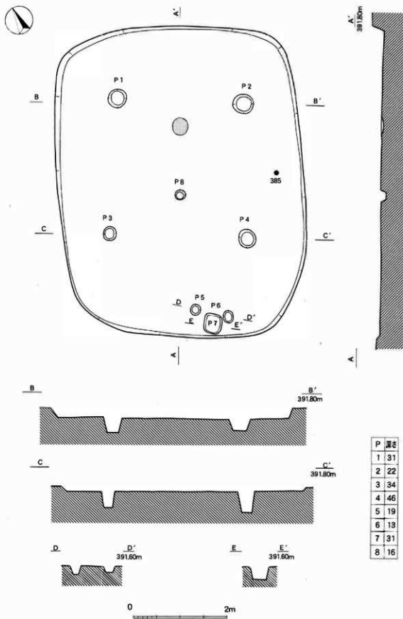
第8图 11号住居址实测图 (1:60)
