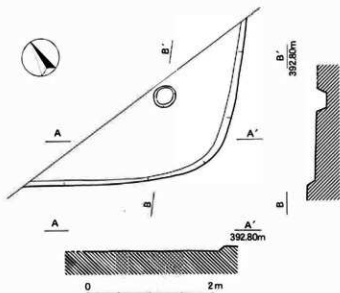
第21図 14号住居址実測図 (1:60)
