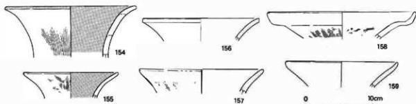
第38図 19号住居址出土土器実測図② (1 : 4)
