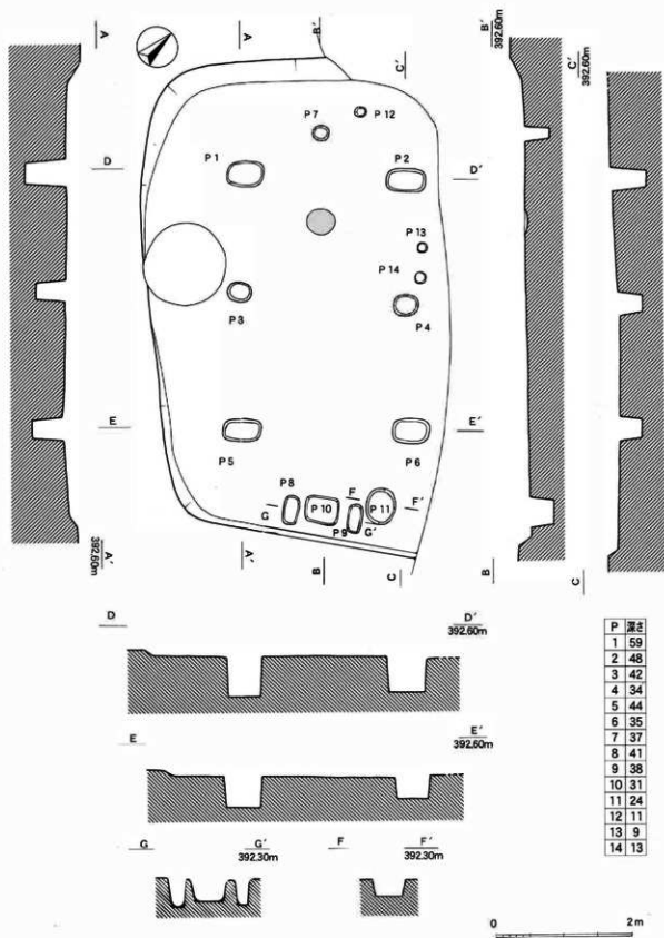
第47图 21号住居址実測图 (1:60)
