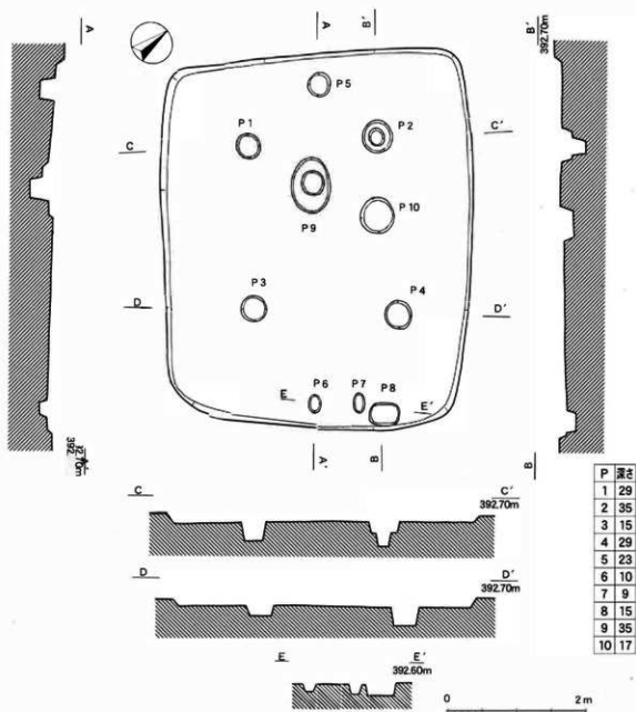
第50図 22号住居址実測図 (1 : 60)
