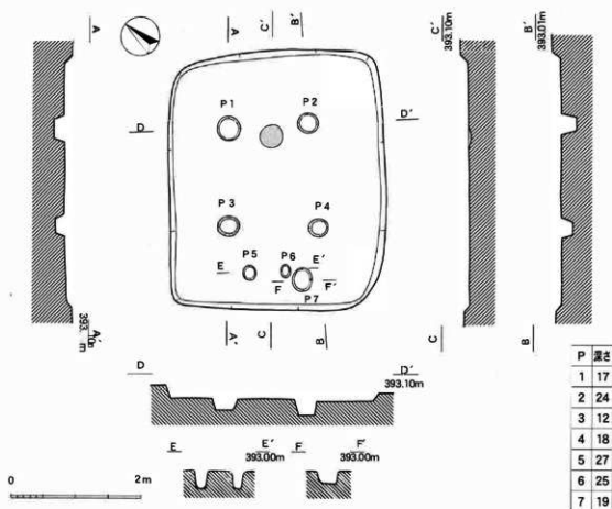
第13図 12号住居址実測図 (1 : 60)
