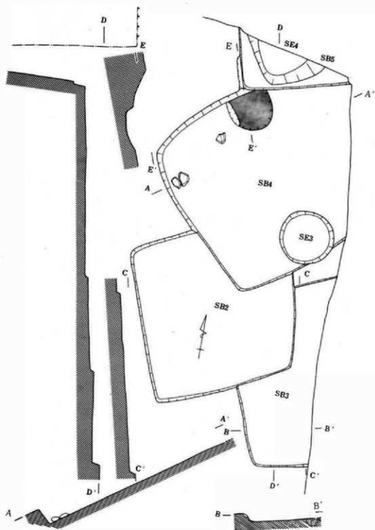
图10 2-5号住址、3·4号井址平面图
