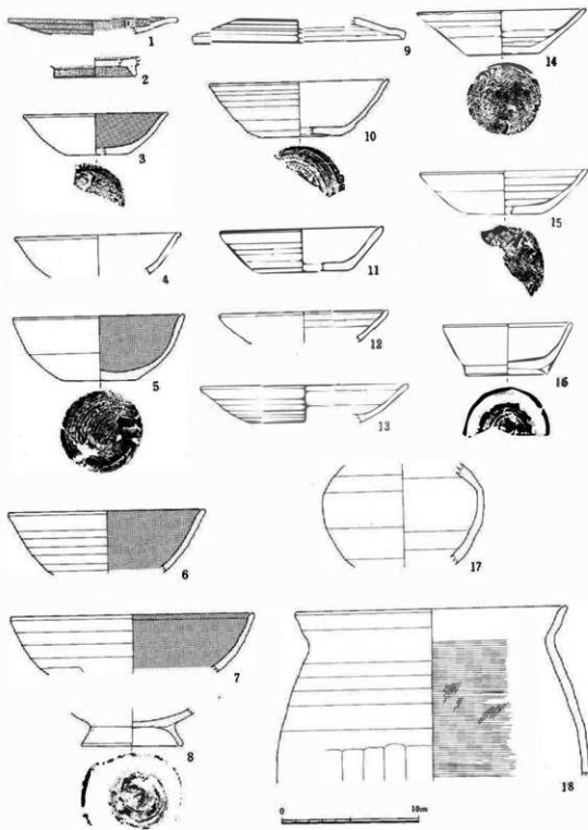
图11 4号住居址出土土器实测图
