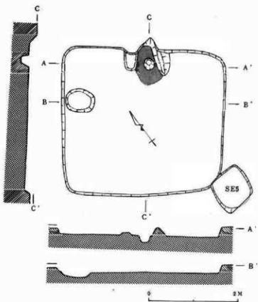
図5 1号住居址実測図
