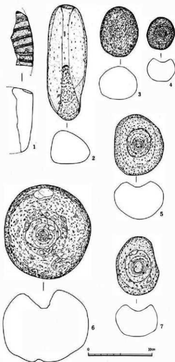
図17 遺構及び遺構外出土石器実測図
