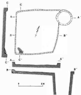
図8 2号住居址、3号井戸址実測図
